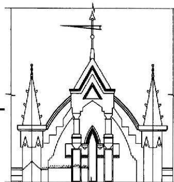
Деталь 1 М 1:50
