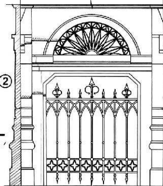
Деталь 2 М 1:50
