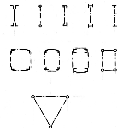
Рисунок 4.2 – Поперечні перерізи ферм: плоскі, коробчасті, трикутні
