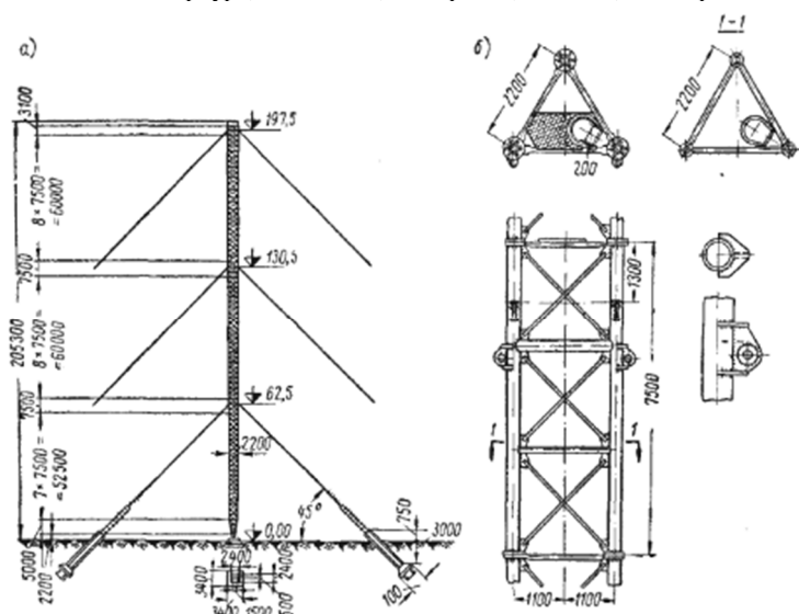
Рисунок 4.21 – Трихгранна трубчата радіощогла: а – загальний вид; б – типова секція
