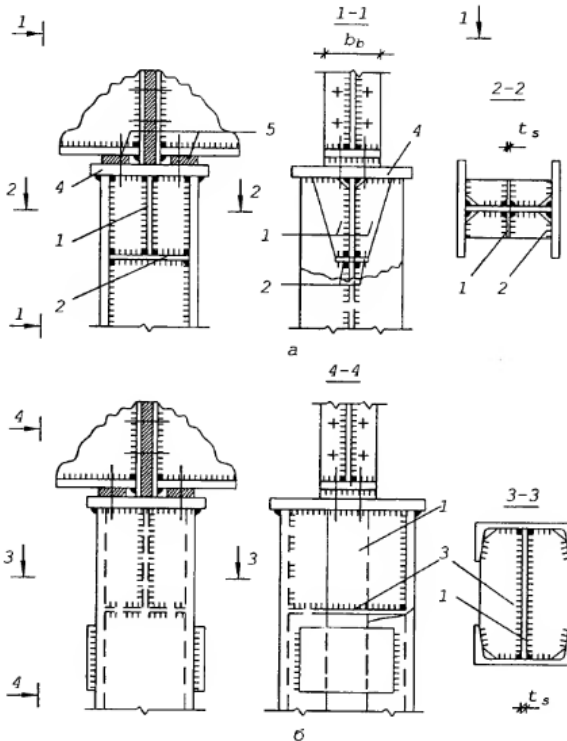
Рисунок 2.20 – Найпоширеніші конструкції оголовків суцільної (а) та наскрісної (б) колони: 1 – вертикальні ребра; 2 – горизонтальні ребра;
