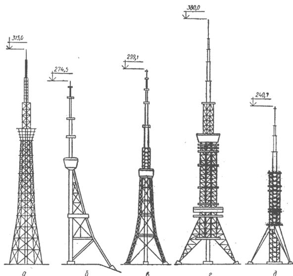
Рисунок 4.20 – Схеми веж телецентрів в містах: а – С. Петербург; б – Тбілісі; в – Среван; г – Київ; д – Харків
