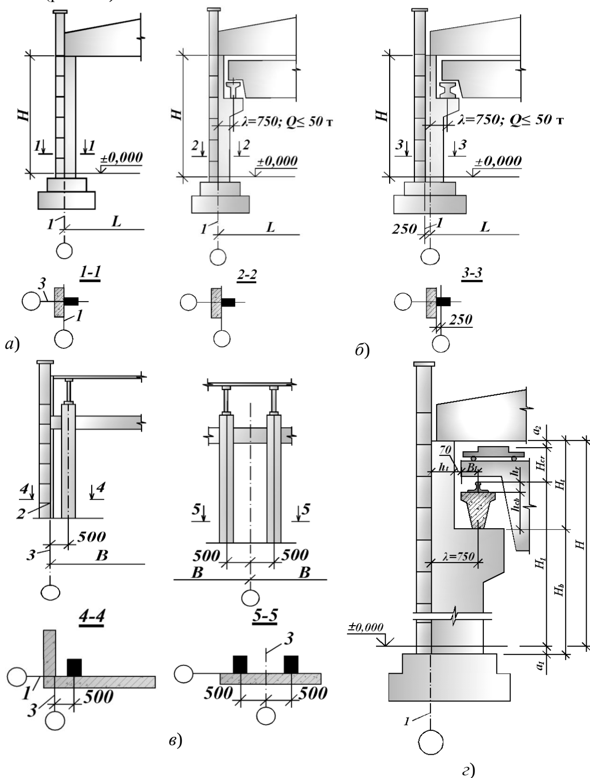
Рисунок 4.2 – Схеми прив'язки колон до координаційних осей (а, б, в) і визначення розмірів колон (г):
