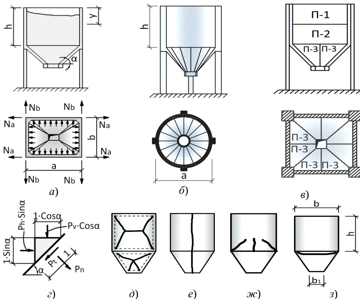
Рисунок 7.7 – Конструкції бункерів та їх розрахункові схеми: а – призматичний монолітний бункер; б – циліндричний монолітний бункер; в – збірний бункер; г – схема зусиль від бічного тиску матеріалу на стінку лійки; д...з – схеми руйнування стінок бункерів
