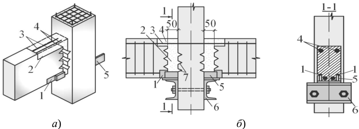
Рисунок 2.31 – Жорсткий безконсольний стик:
