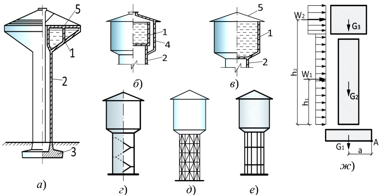
Рисунок 7.6 – Конструкції та розрахункові схеми водонапірних башт:
