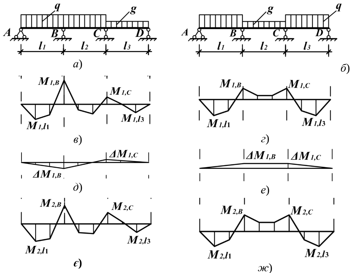
Рисунок 1.4 – Вирівнювання значень згинальних моментів за допомогою додаткових епюр
