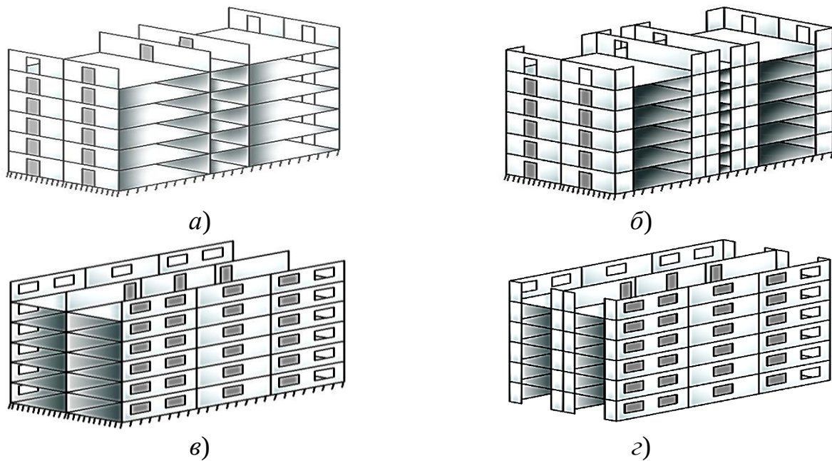
Рисунок 5.20 – Розрахункові схеми крупнопанельних будівель: а, б – з поперечним розташуванням діафрагм без урахування та з урахуванням впливу поздовжніх стін; в, г – з поздовжнім розташуванням діафрагм без урахування та з урахуванням впливу поперечних стін
