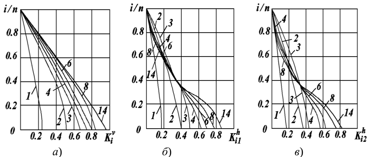
Рисунок 5.22 – Графіки для визначення коефіцієнтів піддатливості: a - K_i^v – від вертикального навантаження; b - K_{i1}^h – від горизонтального рівномірно розподіленого навантаження; v - K_{i2}^h – від горизонтального трикутноподібного навантаження; n – кількість поверхів; i – номер розрахункового поверху; 1...2 – значення величини \mu_n
