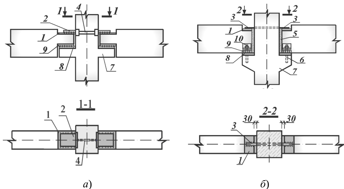
Рисунок 2.30 – Шарнірні стики:
