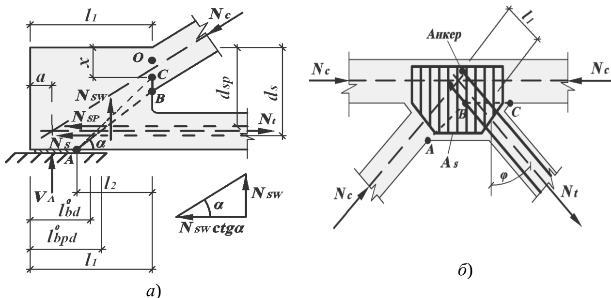
Рисунок 4.15 – Схеми до розрахунку міцності вузлів ферми: а – опорний вузол; б – проміжний вузол
