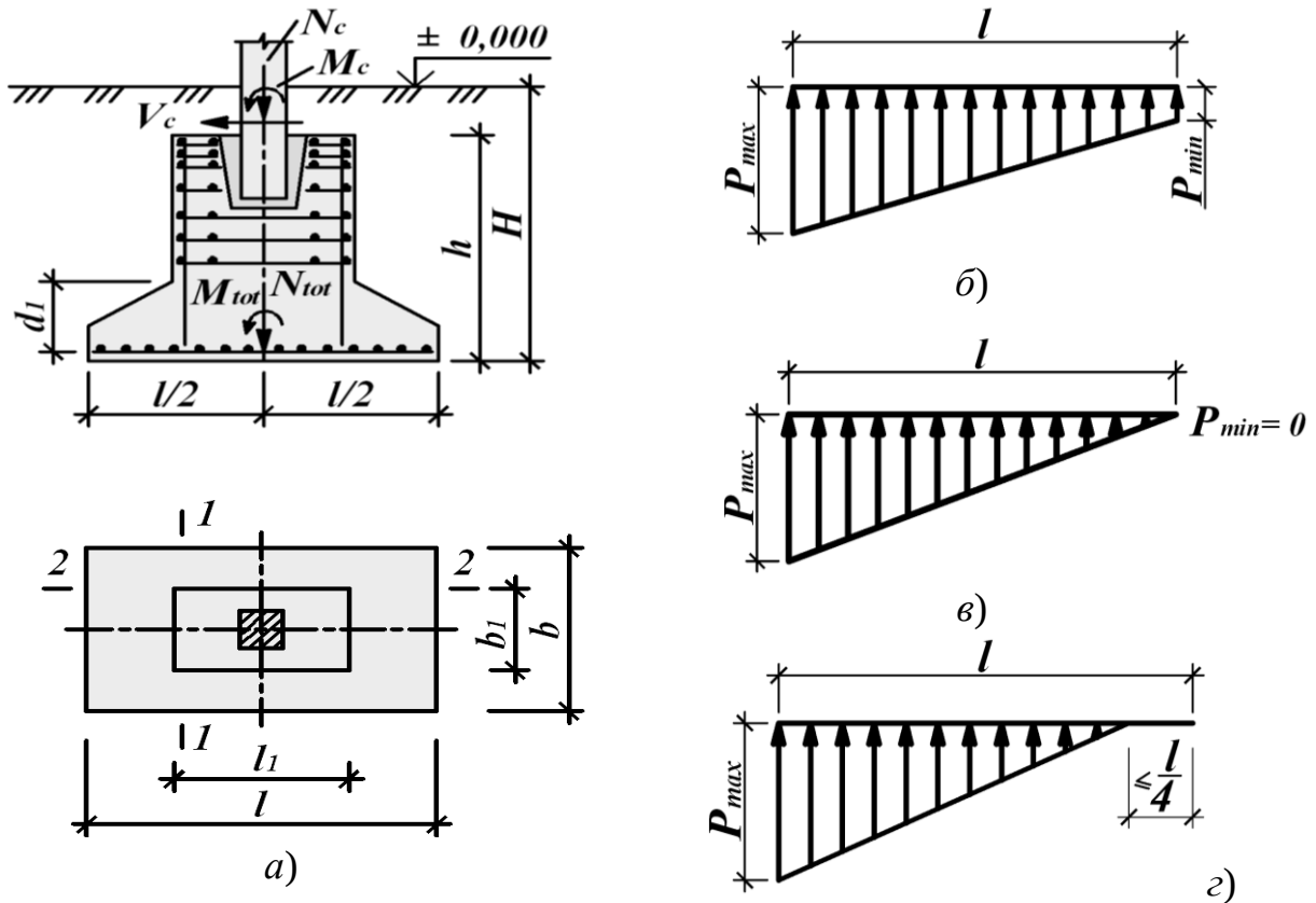
Рисунок 3.4 – Розрахункові схеми з визначення розмірів підшви окремих позацинтрово завантажених фундаментів:
