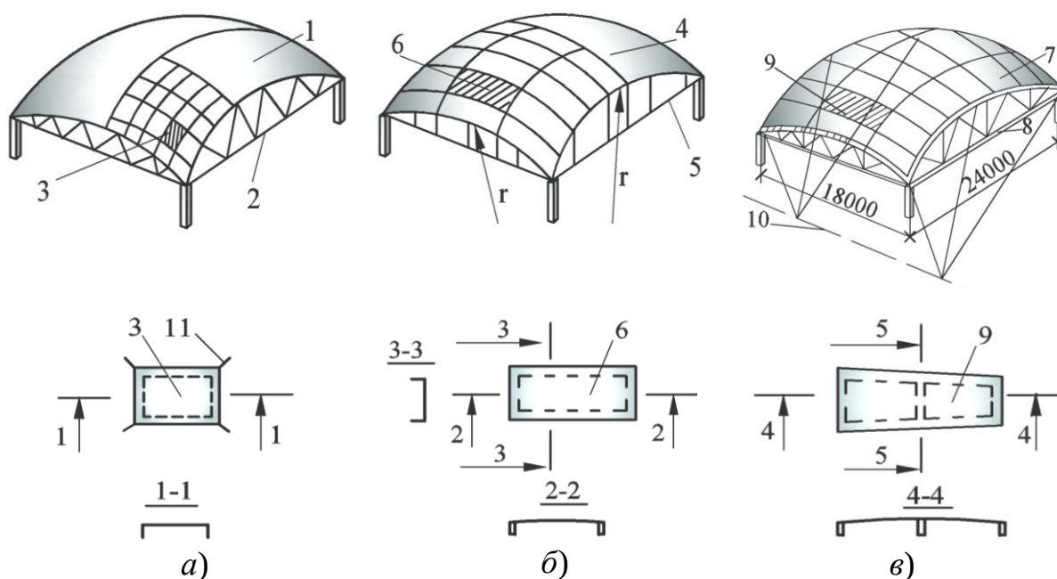
Рисунок 6.4 – Схеми пологих збірних оболонок додатної гаусової кривизни:
