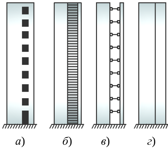
Рисунок 5.18— Розрахункові моделі однов'язевої діафрагми: а – дійсна конструкція; б – дискретно- континуальна модель; в – консольна модель з шарнірними в'язями; г – консольна модель з абсолютно жорсткими в'язями
