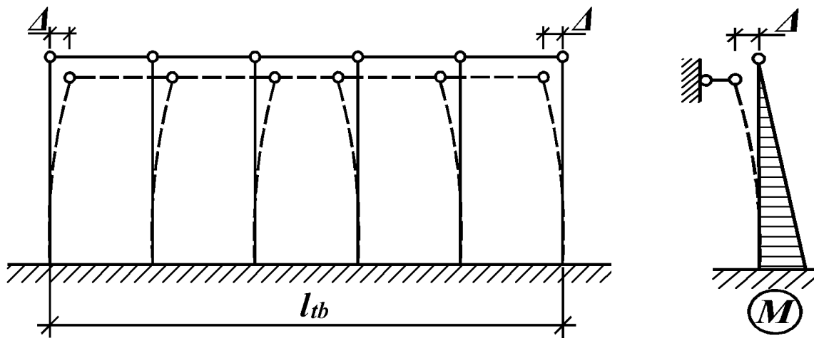
Рисунок 4.3 – Схема деформацій поздовжньої рами від впливу змін температури повітря і усадки бетону
