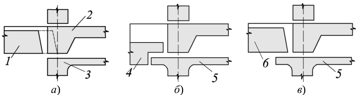
Рисунок 5.13 – Конструкції горизонтальних стиків плит перекриття з об’ємними блоками в панельно-блокових будівлях: а – за допомогою «пальців» у плитах; б, в – на консольні виступи зверху об’ємного блока; 1 – плита перекриття з опорними «пальцями»; 2 – плита підлоги об’ємного блока; 3 – плита стелі об’ємного блока; 4 – плита перекриття з підрізкою на опорі; 5 – об’ємний блок із консолями; 6 – вкорочена плита перекриття
