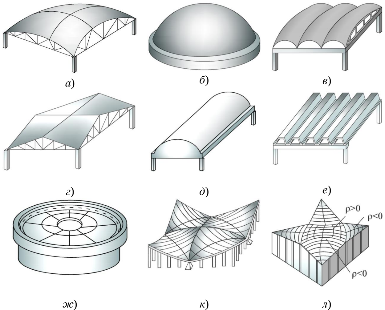
Рисунок 6.2 – Види тонкостінних просторових покриттів:
