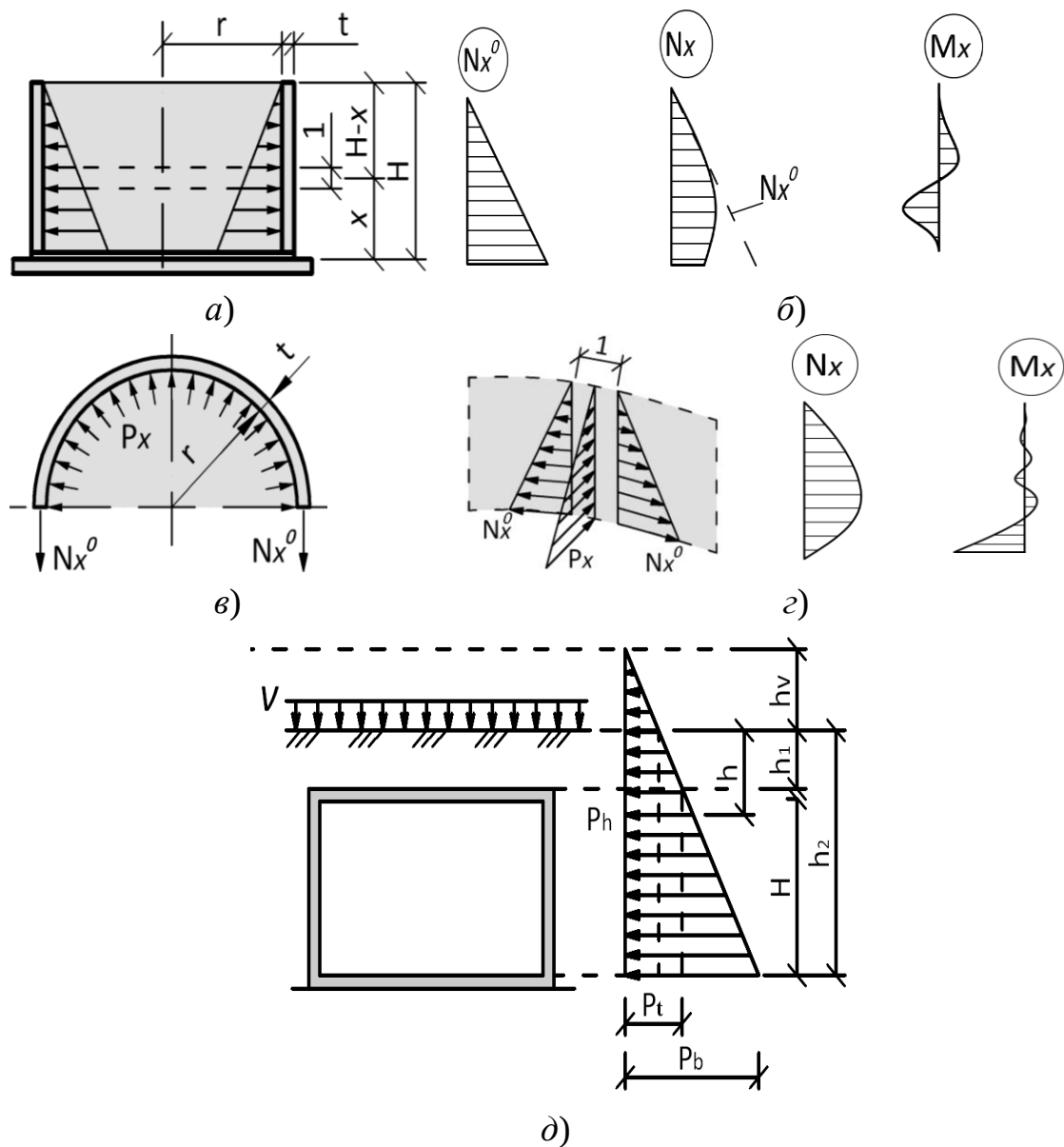
Рисунок 7.2 – До розрахунку циліндричних резервуарів:
