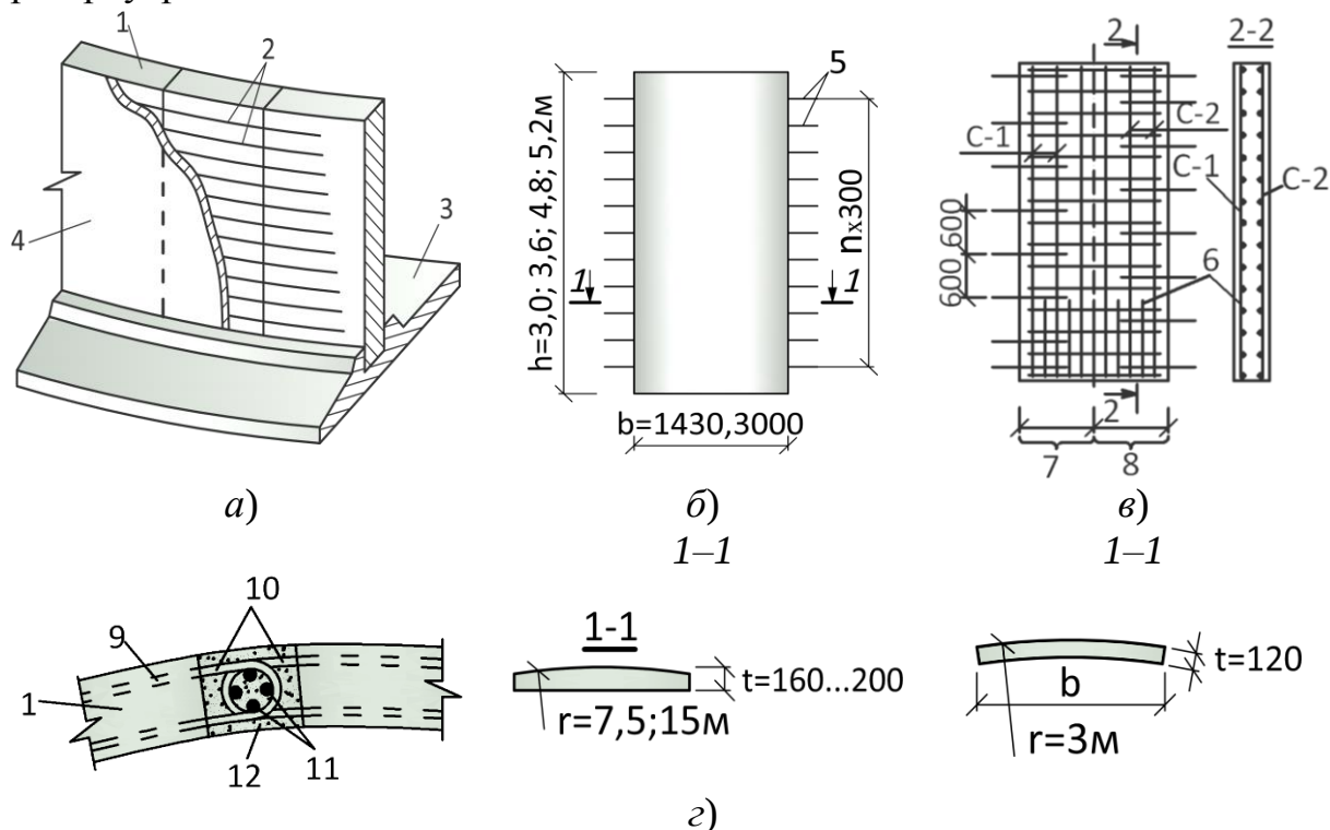
Рисунок 7.3 – Армуння збірних циліндричних резервуарів: а – стінка з попередньо напруженою арматурою; б – загальний вигляд збірної стінової панелі циліндричного резервуару; в – арматура панелі; г – стик панелей з петлевидними випусками арматури; 1 – збірна стінова панель; 2 – кільцева напружена арматура; 3 – днище; 4 – торкрет бетон; 5 – випуски арматури для зварювання панелей; 6 – додаткові стержні; 7 – зовнішня арматурна сітка; 8 – внутрішня арматурна сітка; 9 – кільцева ненапружена арматура панелі; 10 – петлевидні арматурні випуски; 11 – вертикальні арматурні стержні стика; 12 – монолітний бетон стика
