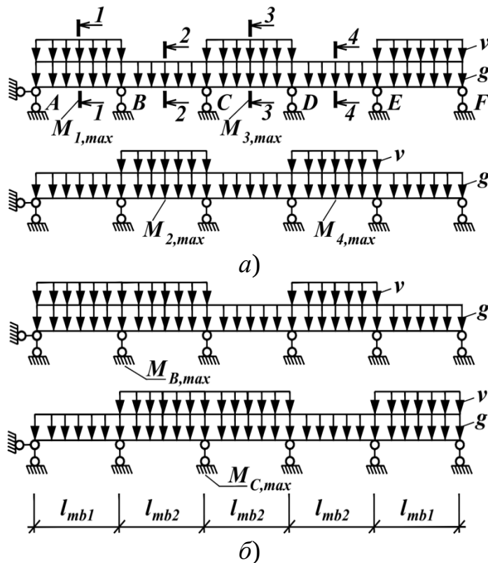
Рисунок 2.28 – Розрахункові схеми нерозрізних ригелів:
