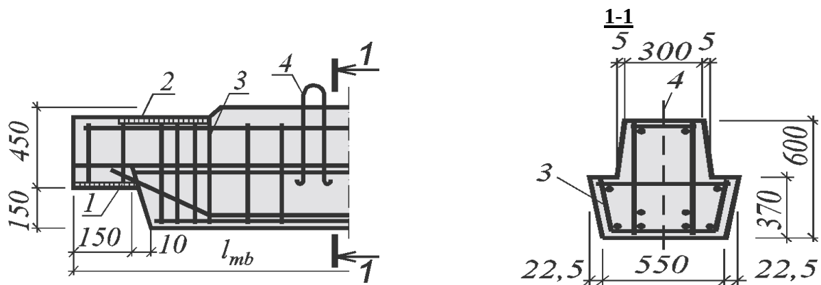
Рисунок 2.29 – Конструкція ригеля з підрізкою на опорі: 1 – опорна закладна деталь для зварювання з консоллю колони; 2 – закладна деталь для монтажної приварювання до колони; 3 – просторовий арматурний каркас; 4 – монтажні петлі
