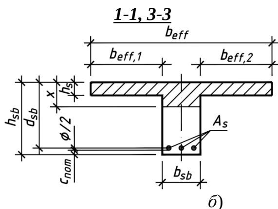
Рисунок 2.12 – До визначення розрахункових прольотів і розмірів поперечного перерізу другорядної балки:
