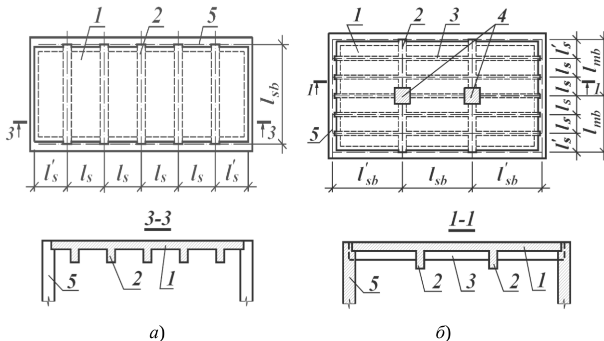
Рисунок 2.2 – Плани монолітних перекриттів:
