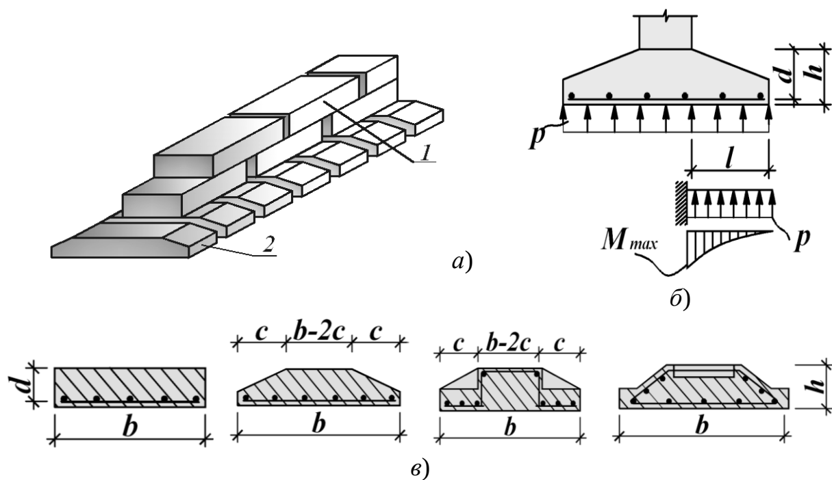
Рисунок 3.5 – Збірний стрічковий фундамент під стіни: а – загальний вигляд; б – схема розрахунку міцності блоків-подушок; в – типи блоків-подушок; 1 – фундаментні блоки; 2 – блоки-подушки
