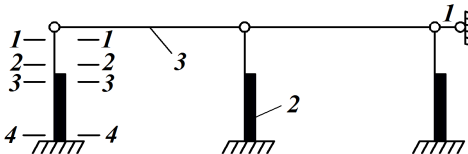
Рисунок 4.9 – Основна система в розрахунках рам методом переміщень:
