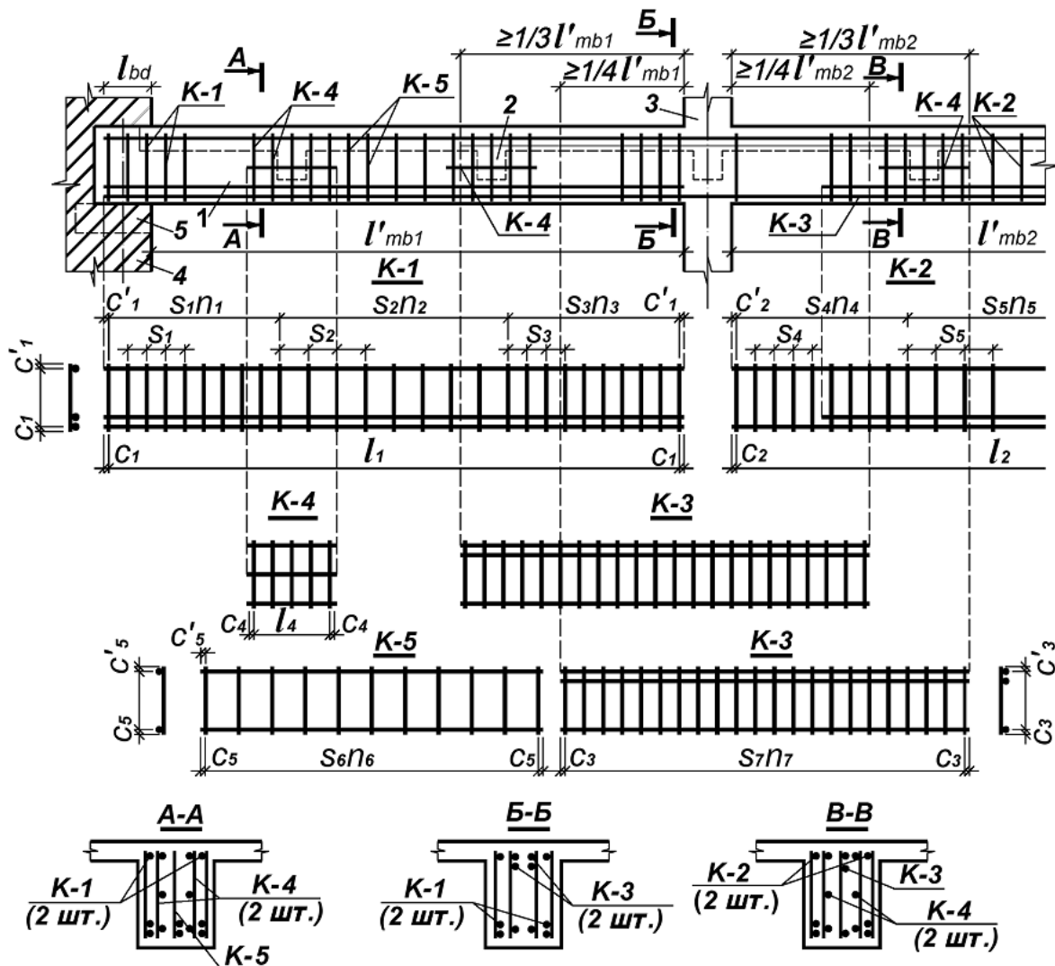
Рисунок 2.18 – Армування головних балок зварними каркасами: 1 – головна балка; 2 – другорядна балка; 3 – колона; 4 – стіна; 5 – опорна подушка; К-І, К-2, К-5 – прольотні каркаси; К-3 – опорний каркас; К-4 – каркаси на ділянці відривання другорядної балки від головної
