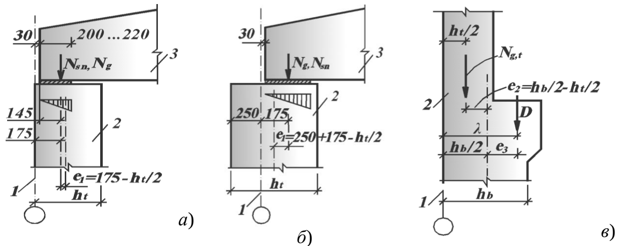
Рисунок 4.8 – До визначення ексцентриситетів зусиль відносно осей колон: а – для верхньої частини колони з нульовою прив'язкою; б – для верхньої частини колони з прив'язкою 250 мм; в – для нижньої частини колони з нульовою прив'язкою 1 – координаційна вісь; 2 – колона; 3 – ригель
