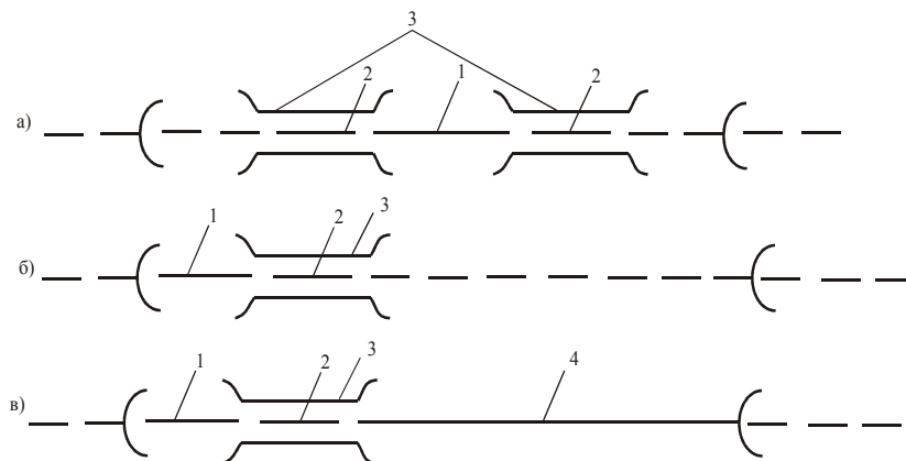
Рисунок 6.2 – Схема ремонту тріснутої або розірваної труби в разі пошкодження: а – середньої частини труби або розтруба; б – хвостової частини; в – усєї труби; 1 – шматок труби без розтруба; 2 – кільце шириною 10 – 12 см; 3 – насувна (ремонтна) муфта; 4 – шматок труби з розтрубом
