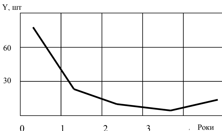
Рисунок 6.4 – Графік зміни питомого числа пошкоджень (Y) сталевих водоводів за роками від початку експлуатації
