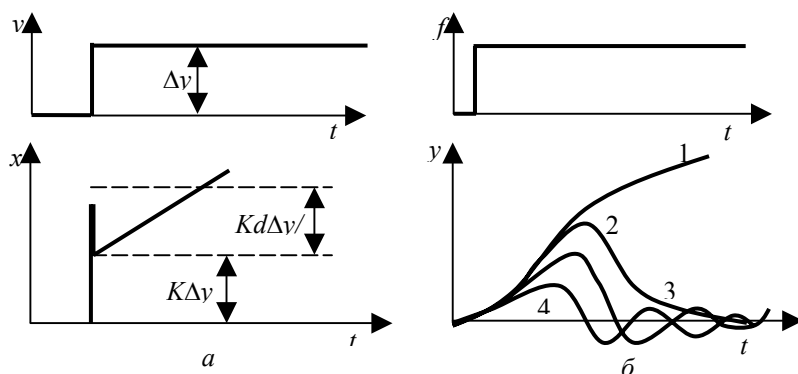
Рис. 5.11. Крива розгону для комплексу технічних засобів, що реалізують ПД-алгоритм керування (а) та результат дії на об'єкт різних алгоритмів керування (б):
