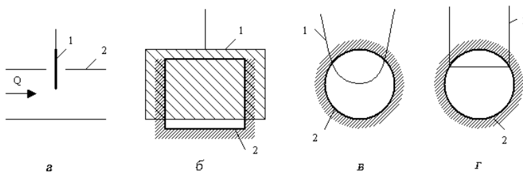
Рис. 5.42. Конструкції шиберів:
