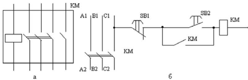
Рис. 3.13. Способи зображення принципових схем: а – суміщений; б – рознесений
