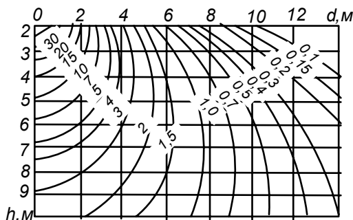
Рис. 4.4. Графік просторових ізолюксів для світильників “Астра-1”, “Астра-11”, “Астра-12”: d – відстань від контрольної точки до проекції світлового центра джерела світла на розрахункову площину
