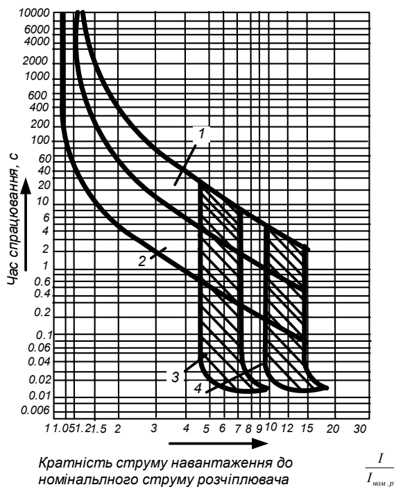
Рис. 6.1. Захисна часострумова характеристика автоматичного вимикача BA51-35:
