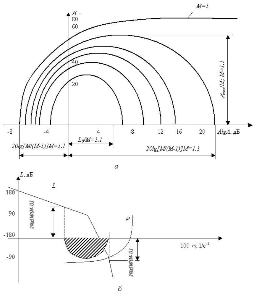
Рис. 5.57. Бажані логарифмічні амплітудно-частотні характеристики цифрових систем: а – для заданого показника коливальності; б – бажана логарифмічна амплітудно-частотна характеристика
