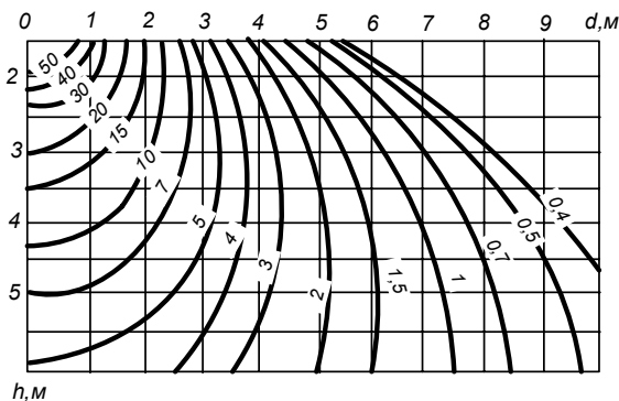
Рис. 4.5. Графік просторових ізолюксів для світильників ППД-100 і ППД-200
