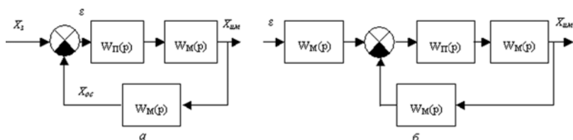
Рис.5.22. Структурно-алгоритмічна схема П-регулятора: а – без додаткового підсилювача; б – з додатковим підсилювачем
