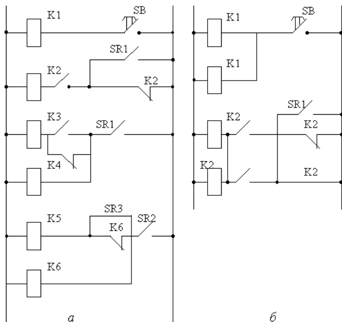
Рис. 8.2. Принципова електрична схема: а – початкова; б – після резервування її елементів
