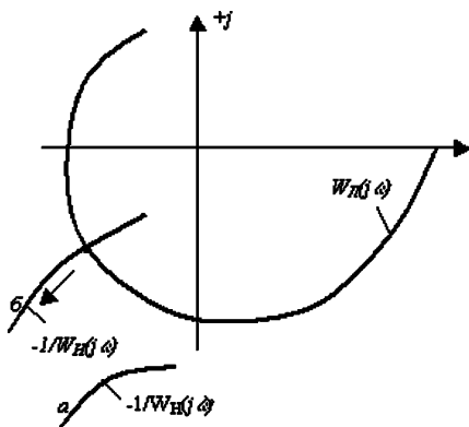
Рис. 5.50. Розташування годографів на комплексній площині: a – для умов, коли в системі не виникають стійкі автоколивання; b – для умов, коли в системі стійкі автоколивання виникають
