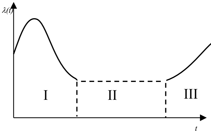
Рис. 8.1 Залежність інтенсивності відмов від часу: I – припрацювання; II – нормальна експлуатація; III – старіння співвідношенням
