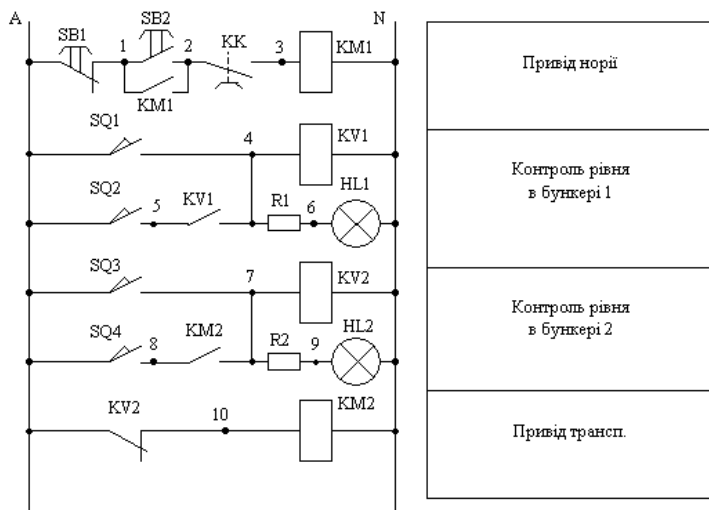
Рис. 3.12. Фрагмент електричної принципової схеми, що виконано рядковим методом з пояснюючими надписами
