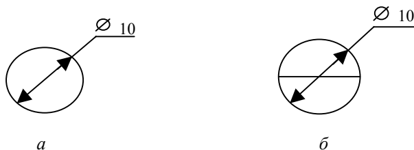
Рис. 3.3. Умовне зображення приладів, встановлених: а – безпосередньо на технологічному обладнанні; б – на щиті керування
