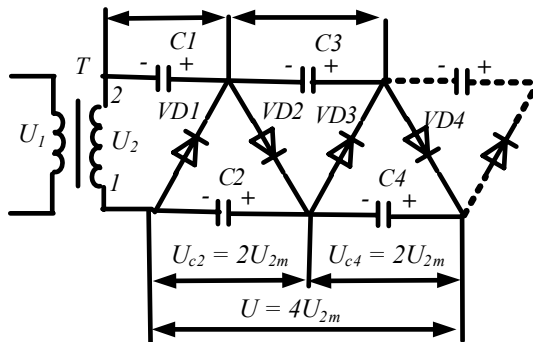
Рис. 4.12. Однонапівперіодна схема множення напруги
