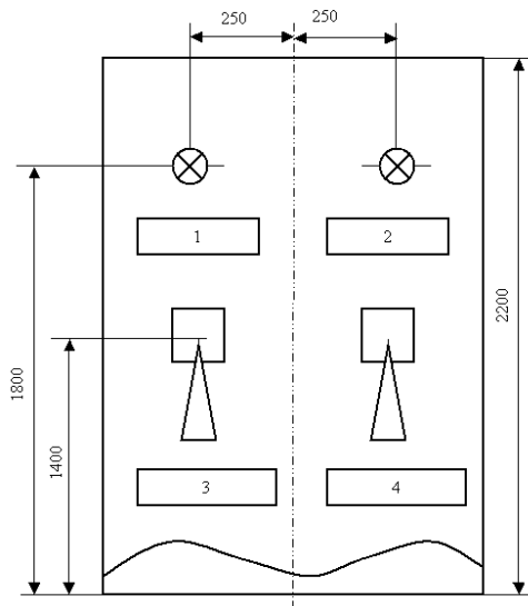
Рис. 7.3. Фрагмент загального вигляду щита керування
