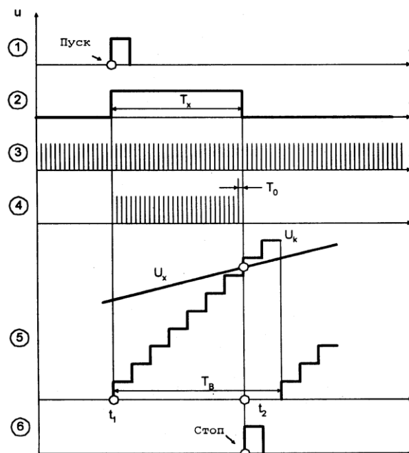
Рисунок 5.18 - Часові діаграми роботи цифрового вольтметра послідовного наближення
