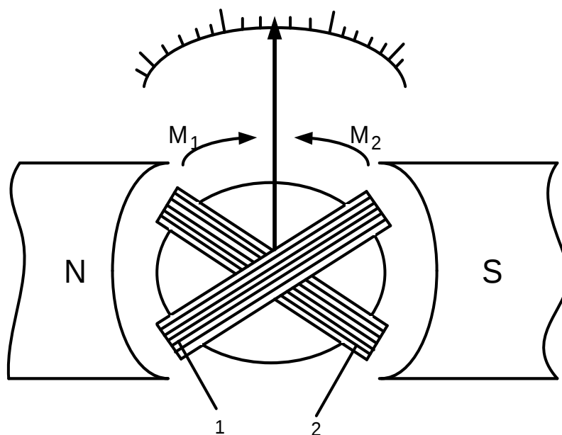
Рисунок 3.3 - Схема вимірювального механізму магнітоелектричного логометра
