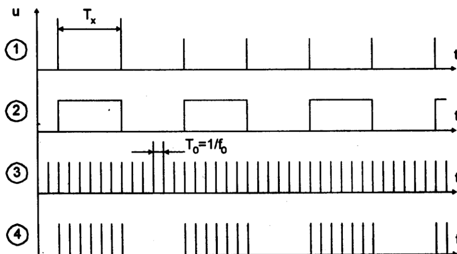
Рисунок 5.6 - Часові діаграми роботи частотоміра миттєвих значень (періодоміра)
