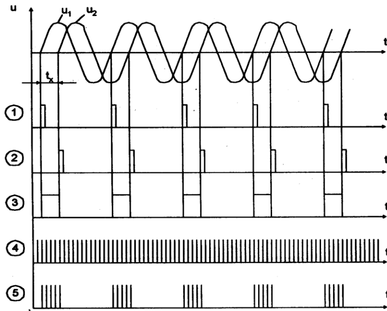
Рисунок 5.10 - Часові діаграми цифрового фазометра миттєвих значень
