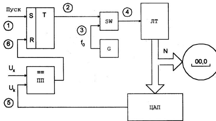
Рисунок 5.17 - Структурна схема вольтметра послідовного наближення
