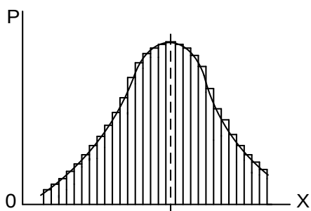
Рисунок 2.2 - Гістограма розподілу
