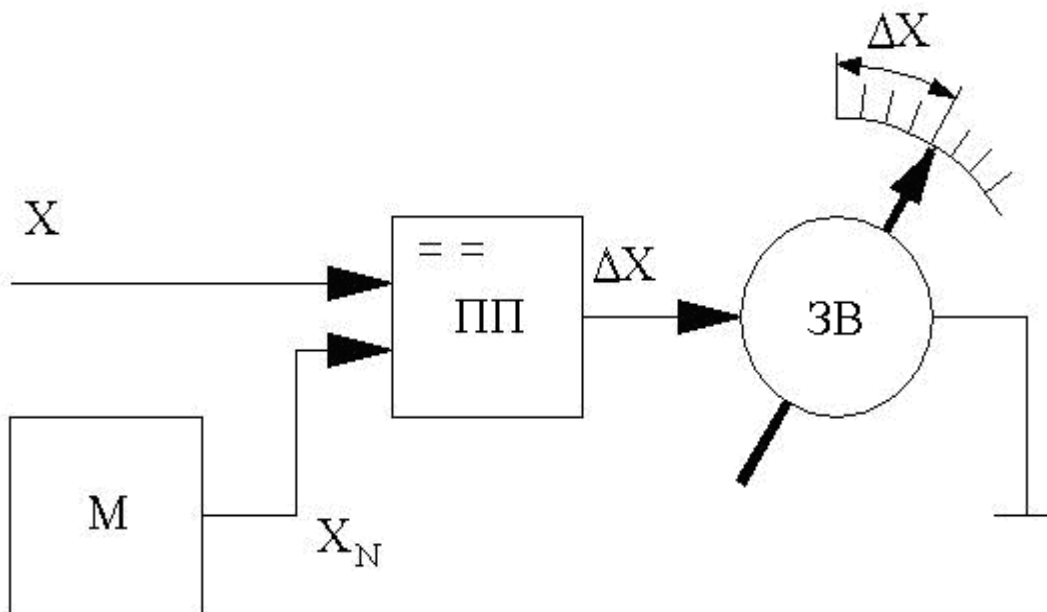
Рисунок 1.5 - Структурна схема диференціального методу
