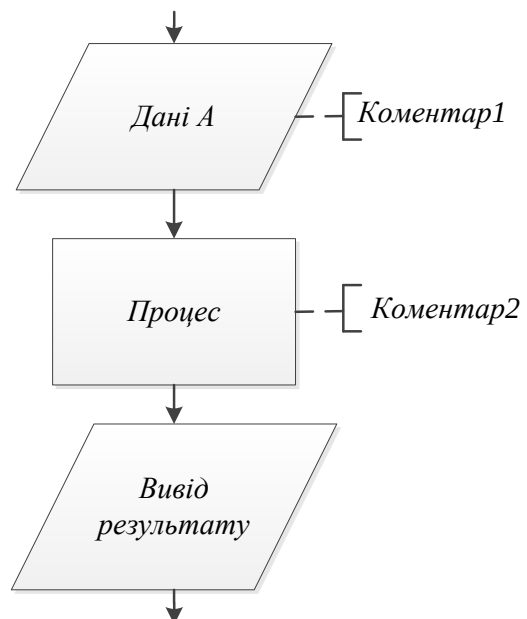
Рис. 1.9. Використання коментарю
