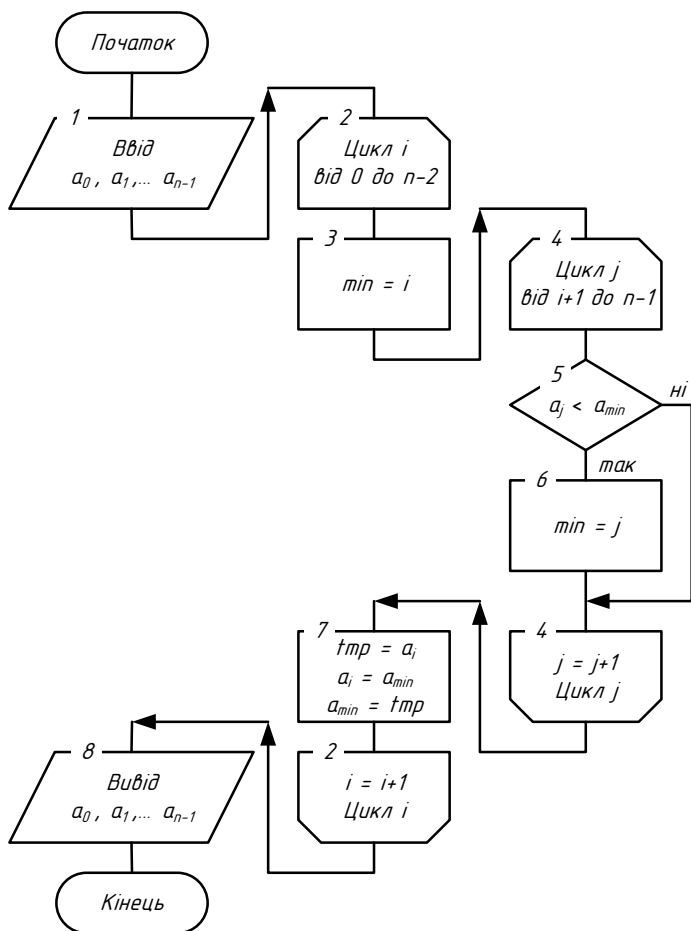
Рис. 0.7 Блок-схема алгоритму сортування вибором
