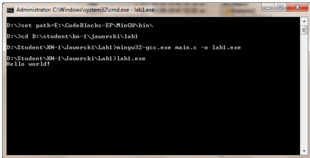
Рис. 1.31 Компіляція та компоновання програми "Hello world!" з допомогою консольних команд операційної системи Windows та компілятора MinGW
