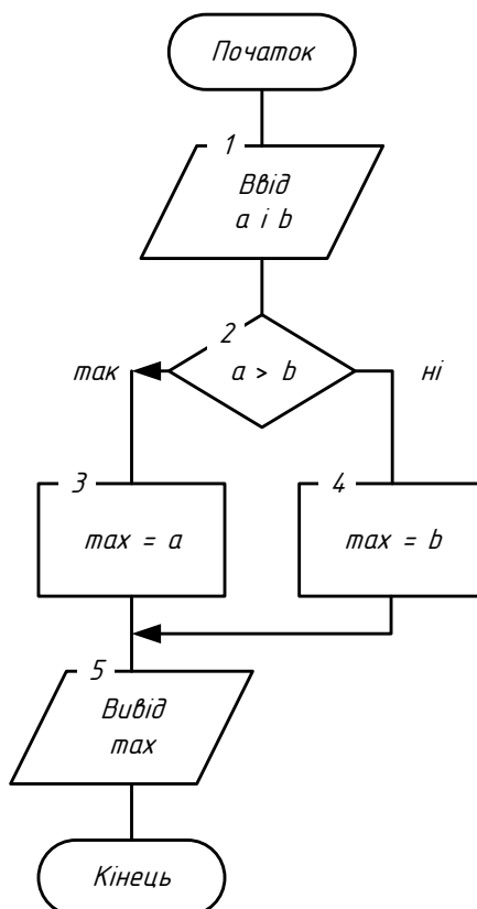
Рис. 0.2 Блок-схема алгоритму з розгалуженням
