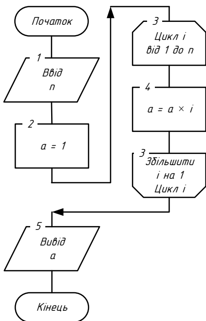
Рис. 0.3 Блок-схема алгоритму циклічної структури
