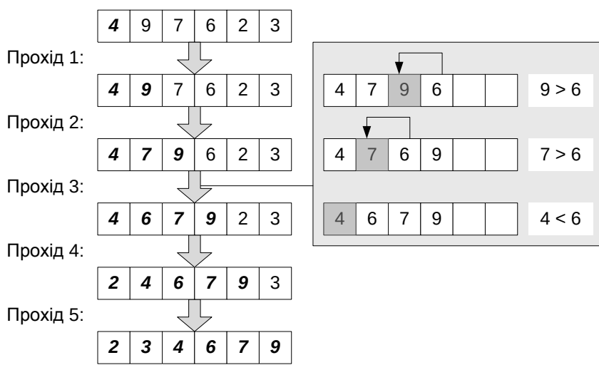
Рис. 0.10 Алгоритм сортування вставками
