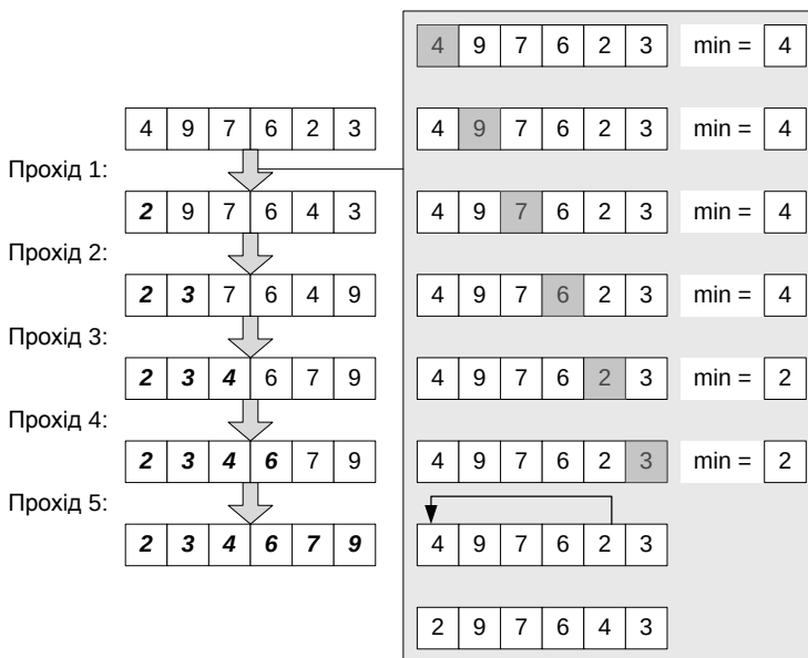
Рис. 0.6 Сортування вибором
