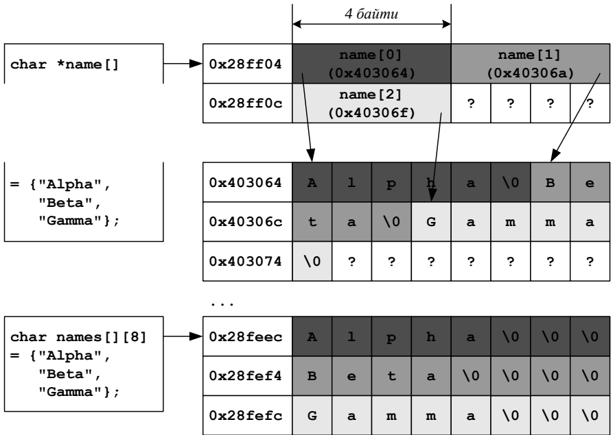
Рис. 6.1 Розміщення рядків символів у пам'яті при ініціалізації
