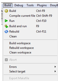
Рис. 1.20 Меню Build
