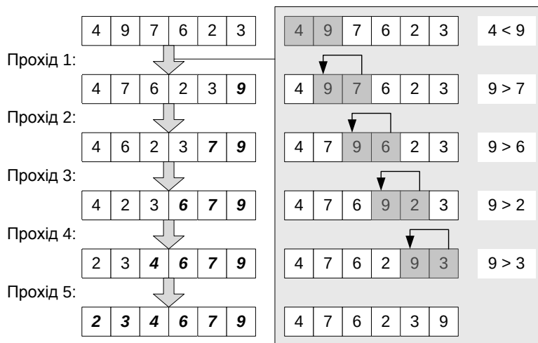
Рис. 0.8 Бульбашкове сортування
