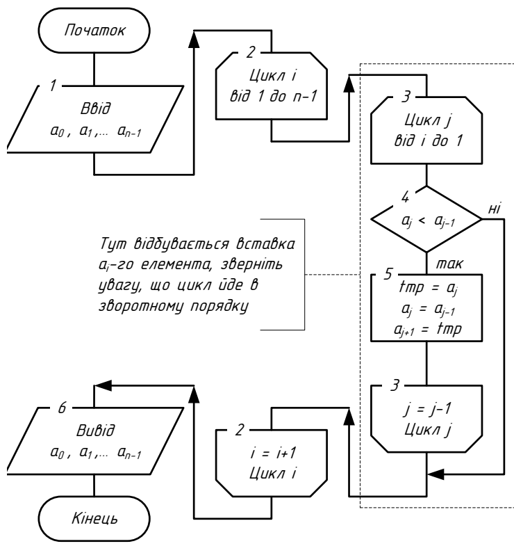
Рис. 0.11 Блок-схема алгоритму сортування вставками
