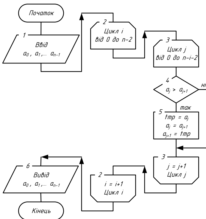
Рис. 0.9 Блок-схема алгоритму бульбашкового сортування
