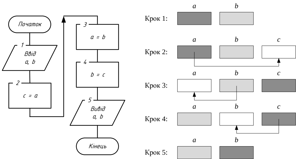
Рис. 0.5 Алгоритм обміну двох змінних місцями
