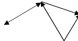
напрямлені дуги, орієнтований граф
