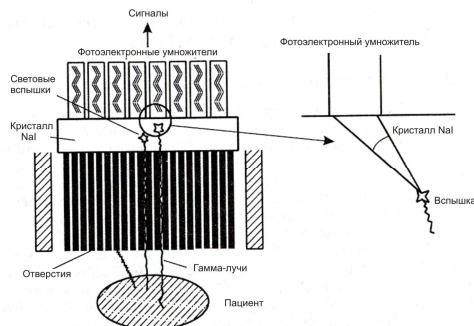
Рис. 31.1. Строение гамма-камеры
