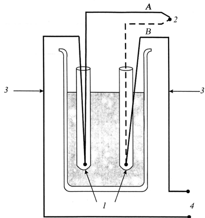
Рис. 9.16. Эффект Зеебека – возникновение термоэлектродвижущей силы (термоз.д.с.) в электрической цепи, состоящей из последовательно соединенных разнородных проводников, контакты которых имеют разную температуру: 1 – опорные спаи; 2 – измерительный спай; 3 – медный проводник; 4 – выход к потенциометру
