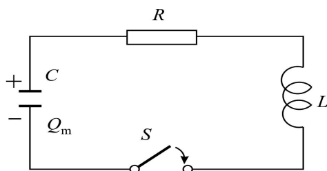
Рис. 15.12. Цепь с сопротивлением, индуктивностью и емкостью
