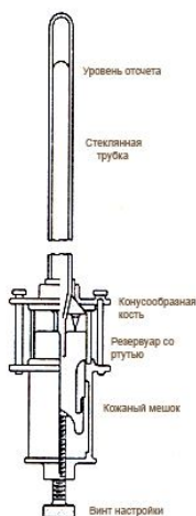
Рис. 4.1. Манометр сифонного типа
