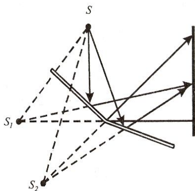
Рис. 20.15. Зеркала Френеля
