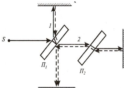
Рис. 20.18. Интерферометр Майкельсона
