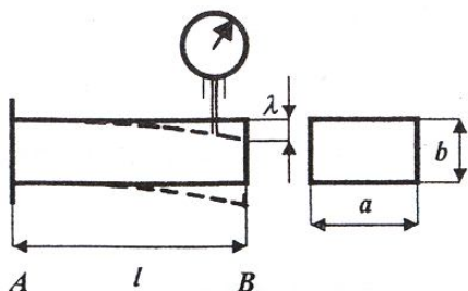
Рис. 2.12. Определение модуля Юнга стержня прямоугольного сечения, один конец которого закреплен
