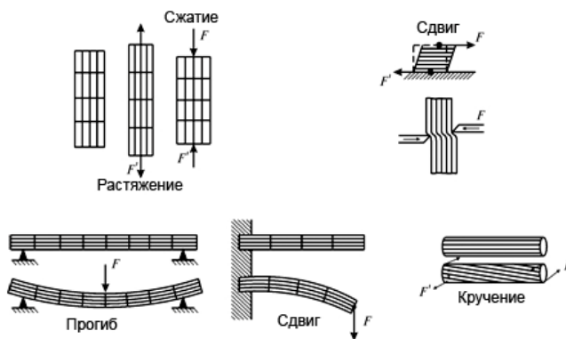
Рис. 2.8. Типы деформаций
