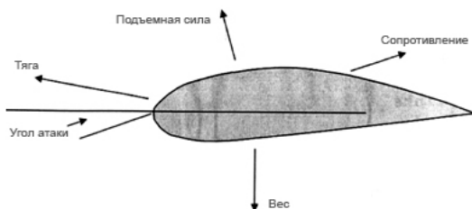
Рис. 4.19. Силы, действующие на крыло птицы
