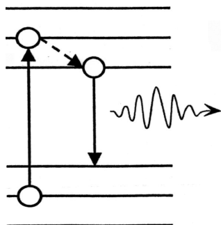
Рис. 28.9. Полупроводниковый лазер, в котором реализуются излучательные переходы между разрешенными энергетическими зонами, а не дискретными уровнями энергии (пояснения в тексте)
