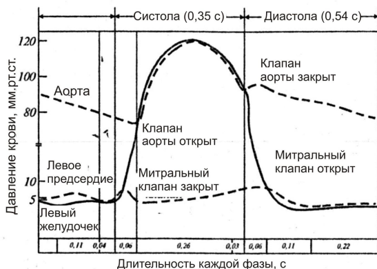
Рис. 4.12. Зависимость давления крови от времени в процессе работы сердца
