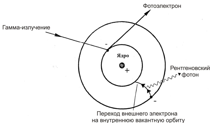
Рис. 30.8. Фотоэлектрическое поглощение
