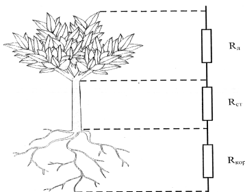
Рис. 9.14. Прохождение воды по растению можно описать последовательным соединением трех проводников, сопротивления которых соответствуют корневой системе ( R_{кор} ), стеблю ( R_{ст} ) и листку ( R_{л} )
