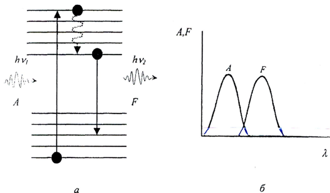
Рис. 27.5. Спектральные свойства молекул: a – поглощение и излучение кванта света молекулой; b – полосы поглощения ( A ) и излучения ( F ) молекулы
