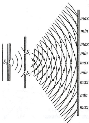
Рис. 20.13. Опыт Юнга
