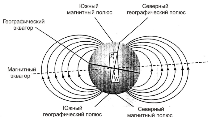
Рис. 15.6. Магнитное поле Земли по форме напоминает поле диполя, центр которого смещен относительно центра Земли, а ось наклонена к оси вращения Земли на 11,5^\circ
