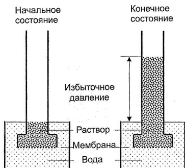
Рис. 7.10. Суммарная диффузия растворителя в раствор через полупроницаемую мембрану
