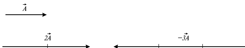
Рис. 1.4. Умножение векторов на скаляр
