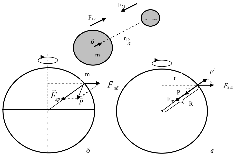
Рис. 2.7. Взаимодействие двух тел: а – взаимодействие двух тел; б – действие сил на тело, находящееся на земной поверхности; в – зависимость веса тела от широты его местонахождения. Здесь: \vec{F}_{гп} – вектор силы гравитации; \vec{F}_{вид} – вектор центробежной силы; \vec{P} – вектор силы тяжести; F_{гп} – сила гравитации; F_{цб} – центробежная сила инерции; P – вес тела, \varphi – географическая широта местонахождения тела, r – радиус вращения тела; R – радиус земного шара.
