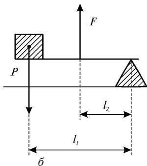
Рис. 2.23. Кости в качестве рычага: а – рычаг, состоящий из плечевой, лучевой костей и мышцы; б – эквивалентная схема рычага: P – груз; F – действующая сила; l_1 и l_2 – плечи рычага
