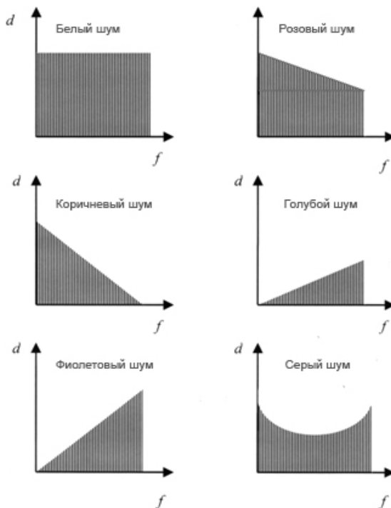
Рис. 6.6. Спектры шумов разных цветов
