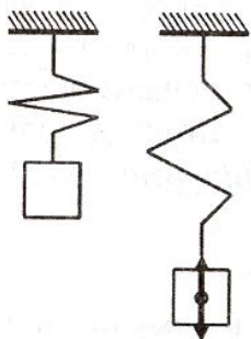
Рис. 5.1. Материальная точка, подвешенная на пружине
