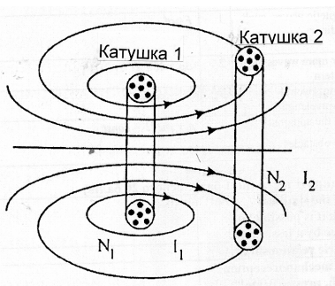
Рис. 15.10. Взаимоиндукция – это явление, в котором проявляется магнитная связь двух или более электрических цепей
