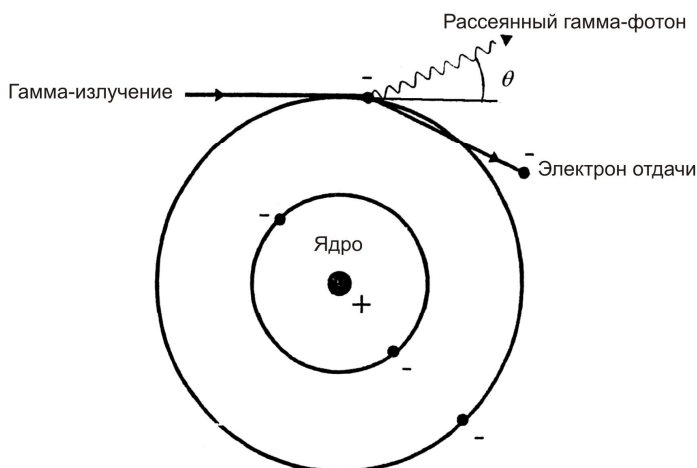
Рис. 30.9. Комптоновский эффект
