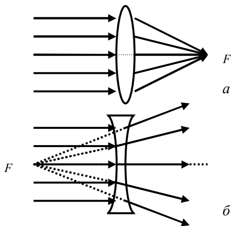
Рис. 20.6. Если линза собирает параллельные лучи в одной точке, она называется собирающей (а); если параллельные лучи, проходящие через линзу, расходятся, она называется рассеивающей (б)
