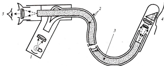
Рис. 20.4. Фиброскоп: 1 – источник света; 2 – внешний световод, обеспечивающий освещение объекта; 3 – внутренний световод, предназначенный для передачи световой информации наблюдателю; 4 – объект; 5 – глаз наблюдателя
