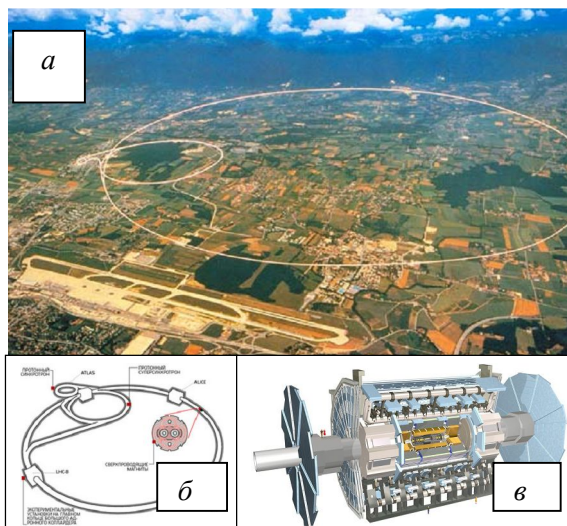
Рис. 15.15. Большой адронный коллайдер: а – ускорительное кольцо БАК (обозначено окружностью белого цвета); на снимке представлен Женевский аэропорт длиной 4 км, позволяющий оценить размер ускорителя CERN; б – расположение протонного синхротрона, протонного суперсинхротрона и детекторов; в – детектор ATLAS (от англ. A Toroidal LHC ApparatuS).
