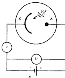
Рис. 20.33. Схема экспериментального прибора, с помощью которого наблюдают явление фотоэффекта: А – анод, К – катод
