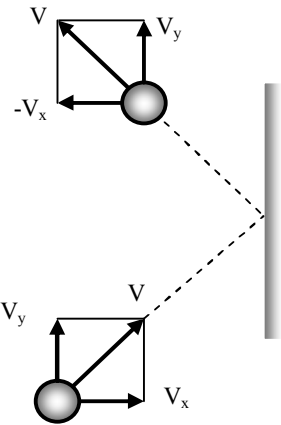
Рис. 7.1. Движение молекулы со скоростью \vec{v} внутри контейнера и упругое столкновение ее со стенкой контейнера, вследствие чего компонента v_x изменяет направление, тогда как направления компонентов v_y и v_z не изменяются
