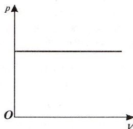
Рис. 7.3. График изобарного процесса в координатах ( p, V )
