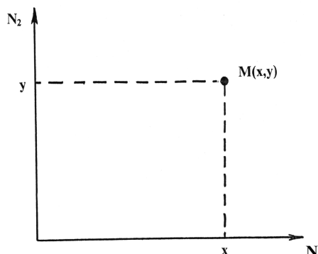
Рис. 5.13. Фазовая плоскость
