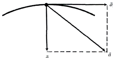
Рис. 2.4. Полное ускорение точки во время криволинейного движения
