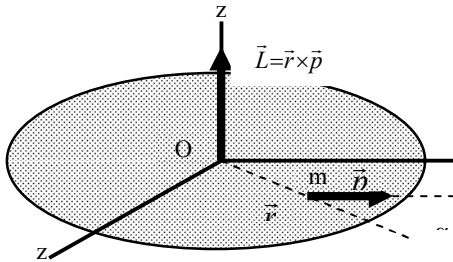
Рис. 2.18. Модуль вектора момента импульса , где \vec{r} – радиус-вектор, проведенный от точки O до материальной точки m ; \vec{p} = m\vec{v} – вектор импульса этой точки; \alpha – угол между векторами \vec{r} и \vec{p}
