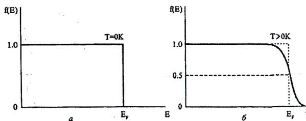
Рис. 28.2. График зависимости функций распределения Ферми-Дирака f(E) от энергии E : a – для T = 0 К; b – для T > 0 К
