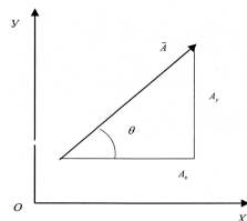
Рис. 1.5. Деление векторов на скаляр Рис. 1.6. Проекции вектора
