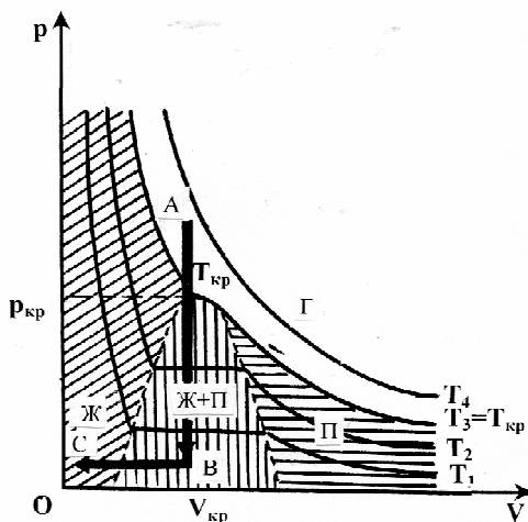
Рис. 7.6. Изотермы реального газа (пояснения в тексте)
