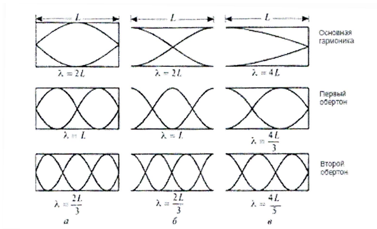
Рис. 6.3. Стоячие волны в трубе: а – закрытой с обоих концов; б – открытой с обоих концов; в – закрытой с одного конца
