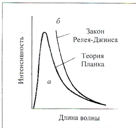
Рис. 20.37 – Сравнение спектра излучения абсолютно черного тела, полученного экспериментально ( а ), с теоретической кривой спектральной зависимости излучения абсолютно черного тела ( б ), описываемой законом Рэлея-Джинса.
