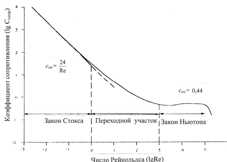
Рис. 4.17. Зависимость коэффициента общего сопротивления C_{con} частицы от числа Рейнольдса Re
