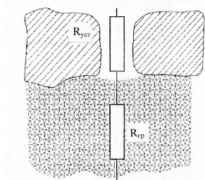
Рис. 9.13. Общее сопротивление устьиц и граничного слоя воздуха
