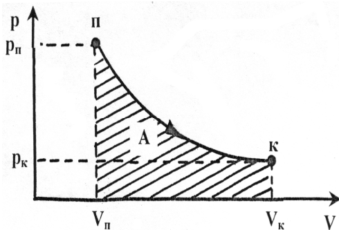
Рис. 8.9. Работа, которую выполняет газ при расширении
