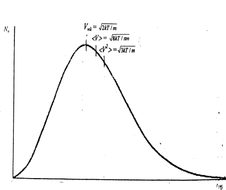
Рис. 7.5. Распределение молекул N_v по скоростям. Здесь: v_{nb} – наиболее вероятная скорость; \langle v \rangle – средняя арифметическая скорость; \langle v^2 \rangle – средняя квадратичная скорость молекул
