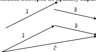
Рис. 1.2. Сложение векторов по правилу треугольника
