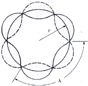
Рис. 24.1. Все возможные состояния электрона как совокупность стоячих волн, каждая из которых имеет свою длину, скорость и энергию
