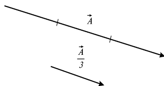
Рис. 1.5. Деление векторов на скаляр Рис. 1.6. Проекции вектора
