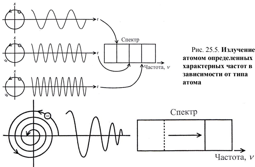
Рис. 25.6. Постепенное изменение частоты излучения вследствие изменения размеров атома во время излучения согласно классической теории
