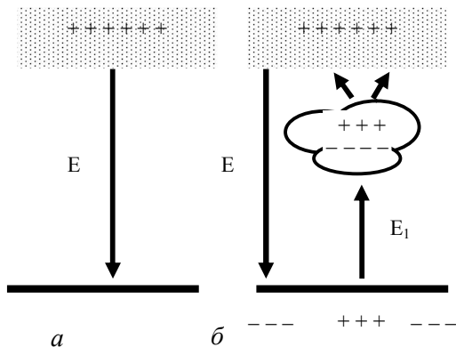
Рис. 10.4. Электрическое поле, образуемое между ионосферой и земной поверхностью: а – при отсутствии грозового облака; б – при наличии грозового облака
