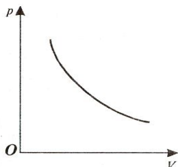
Рис. 7.2. График изотермического процесса в координатах ( p, V )
