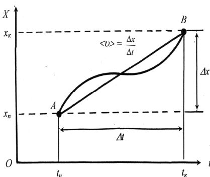
Рис. 2.2. Средняя скорость движения точки
