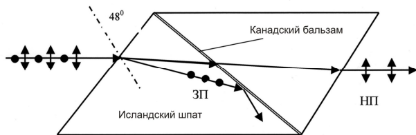
Рис. 20.31. Анизотропия преломления (двойное лучепреломление)
