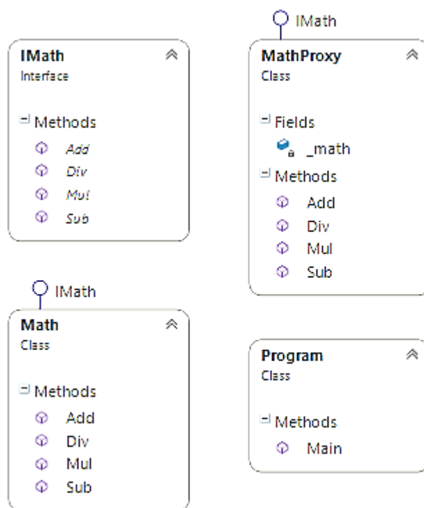
Рис. 6.9. Приклад реалізації шаблону "Замісник"
