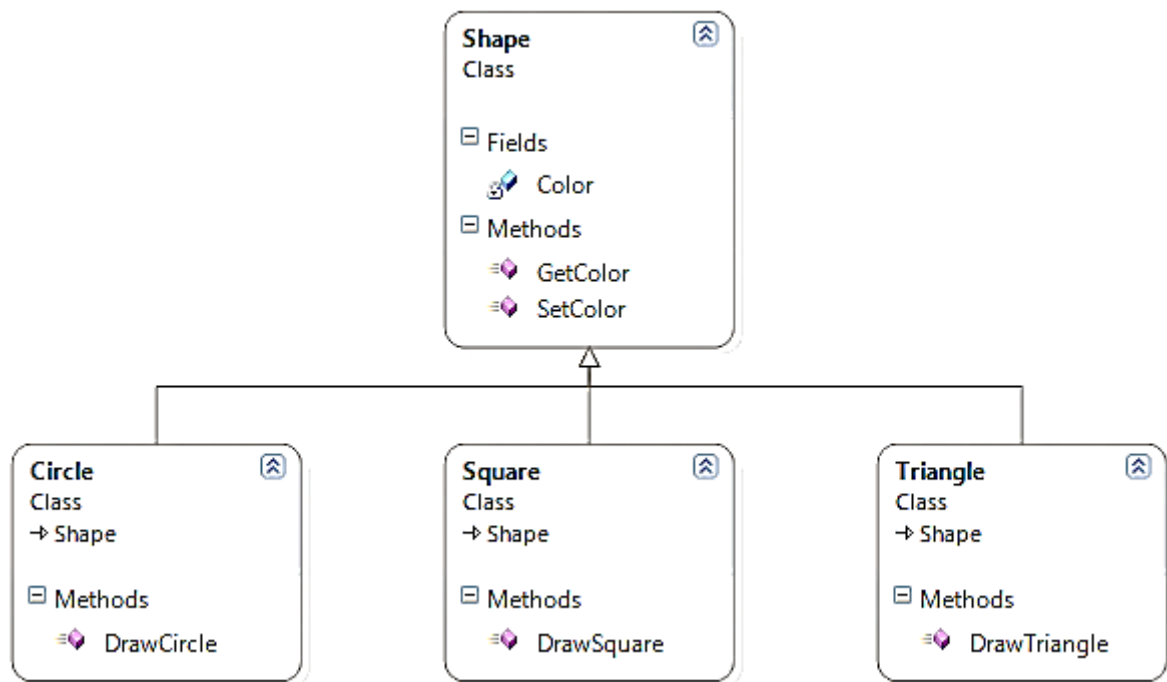
Рис. 6.3. Порушення принципу заміщення Барбари Лісков
