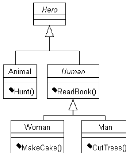
Рис. 5.2. UML-діаграма класів
