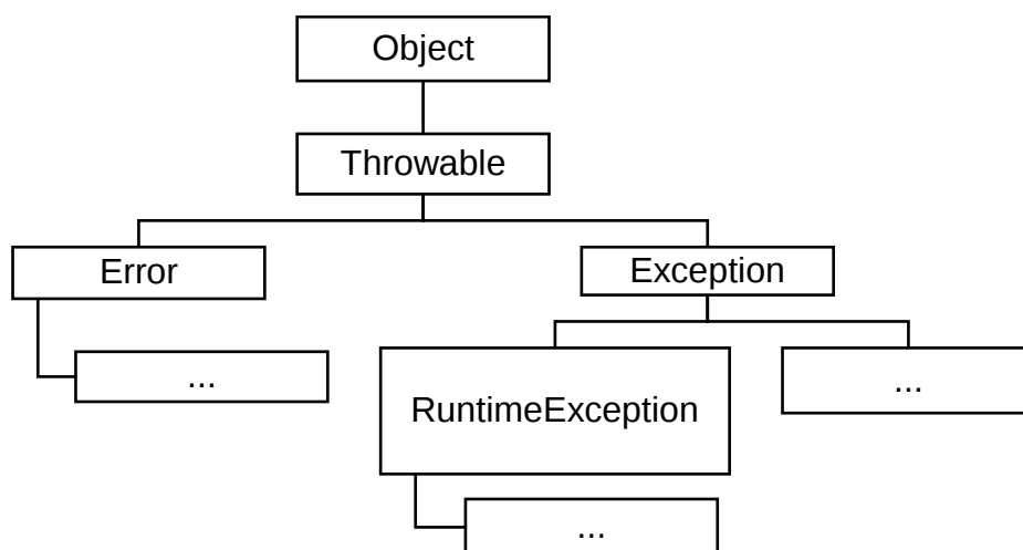
Рис. 8.1. Базові класи системи обробки винятків Java SE
