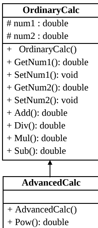
Рис. 3.3. Діаграма класів
