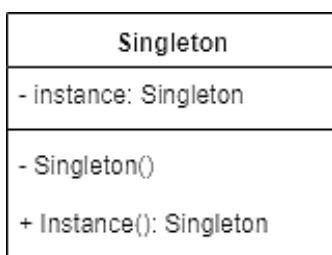
Рис. 6.7. Шаблон "Одинак"
