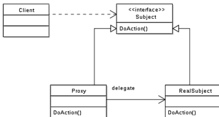
Рис. 6.8. Шаблон "Замісник"
