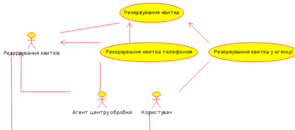
Рис. 10. Діаграми послідовностей
