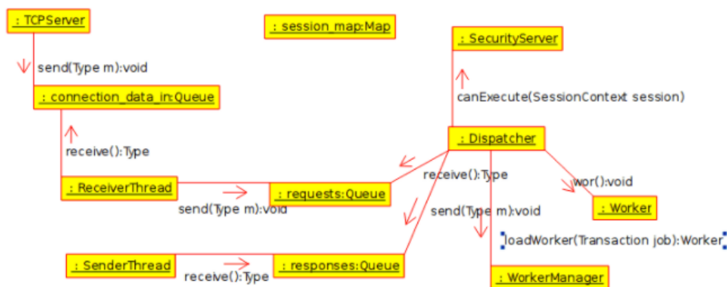
Рис. 11. Діаграми співпраці
