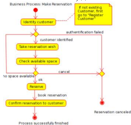
Рис. 13. Діаграми діяльності
