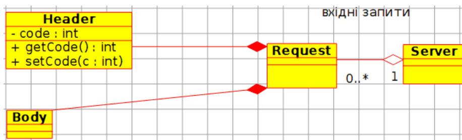
Рис. 3. Діаграми класів
