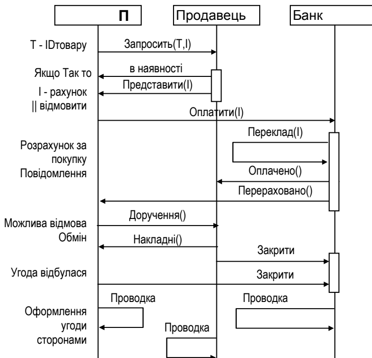
Рис. 7.11. Сценарій торгової операції по безготівковому розрахунку.
