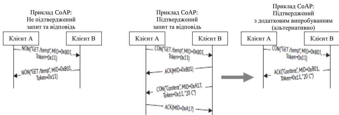
Рис. 3.33. Повідомлення CoAP NON та CON
