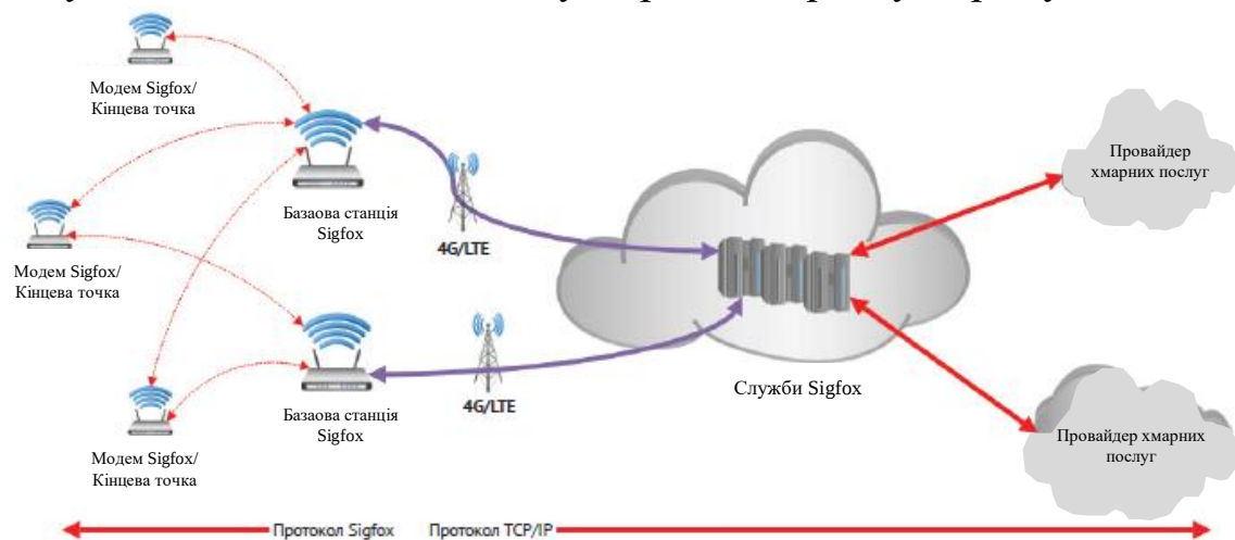
Рис. 3.23. Топологія Sigfox.
