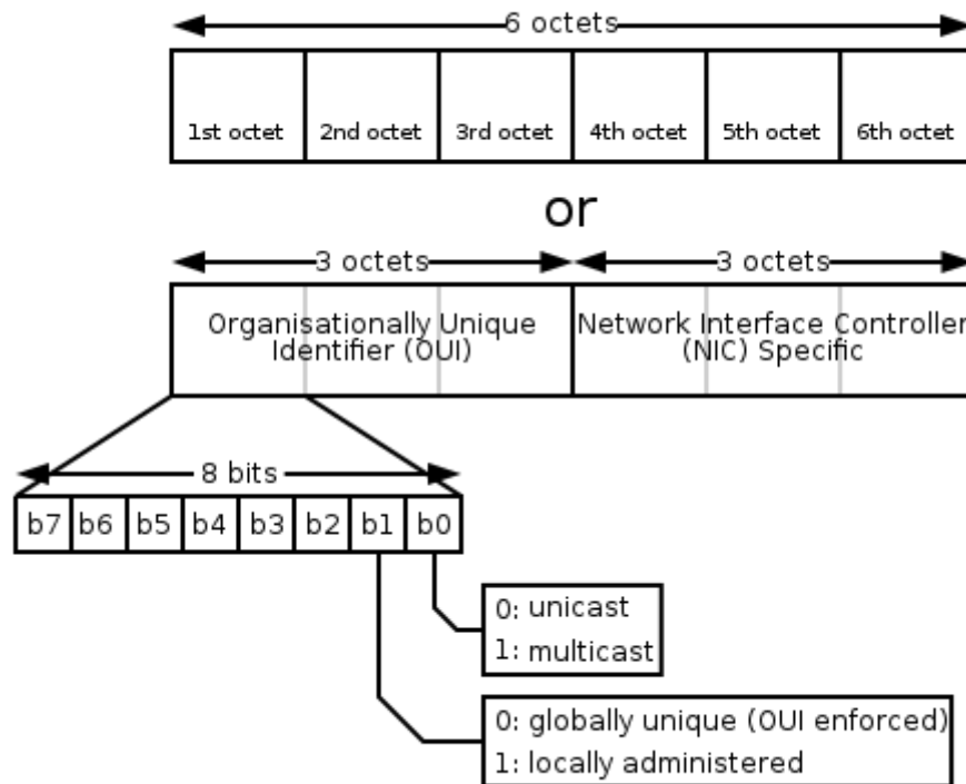
Рис. 2.1. Структура MAC-адреси
