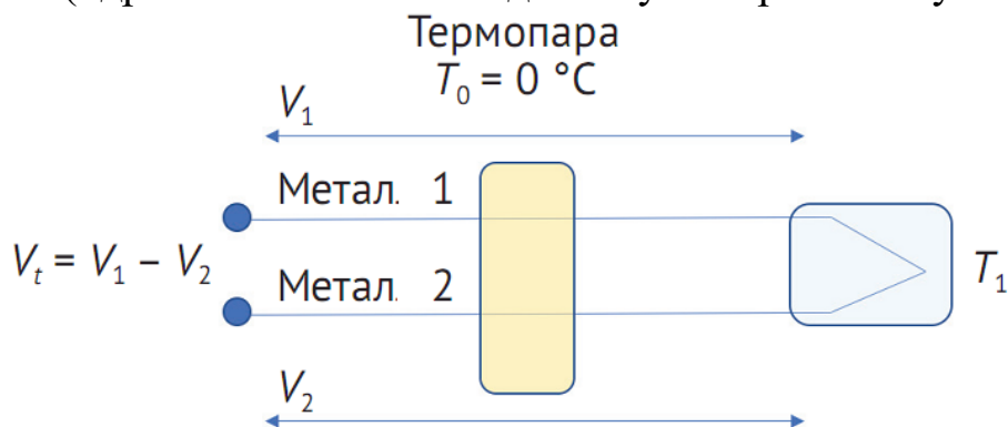
Рис. 2.13. Блок-схема вимірювання температури за допомогою термопари [1]
