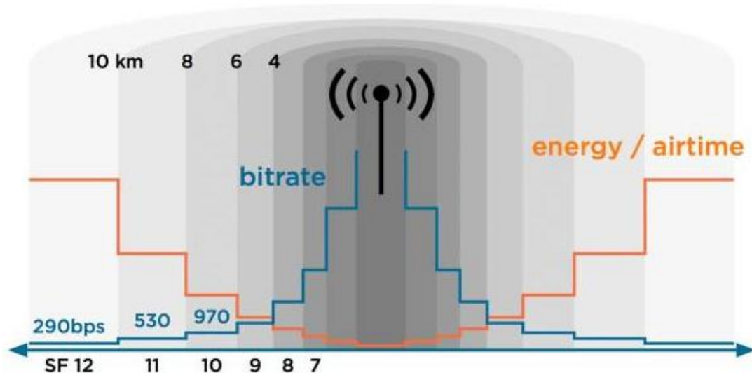
Рис. 3.20. Адаптивна швидкість передачі даних в LoRaWAN мережах
