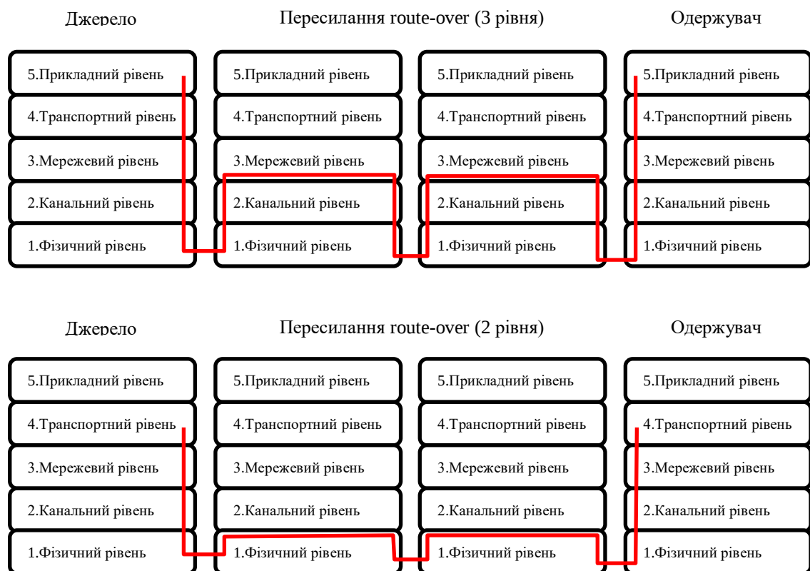
Рис. 3.13. Пересилання пакетів mesh-under та route-over
