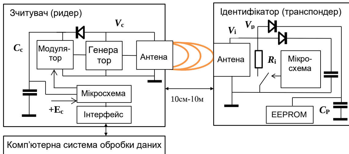
Рис. 2.8. Структура RFID-системи
