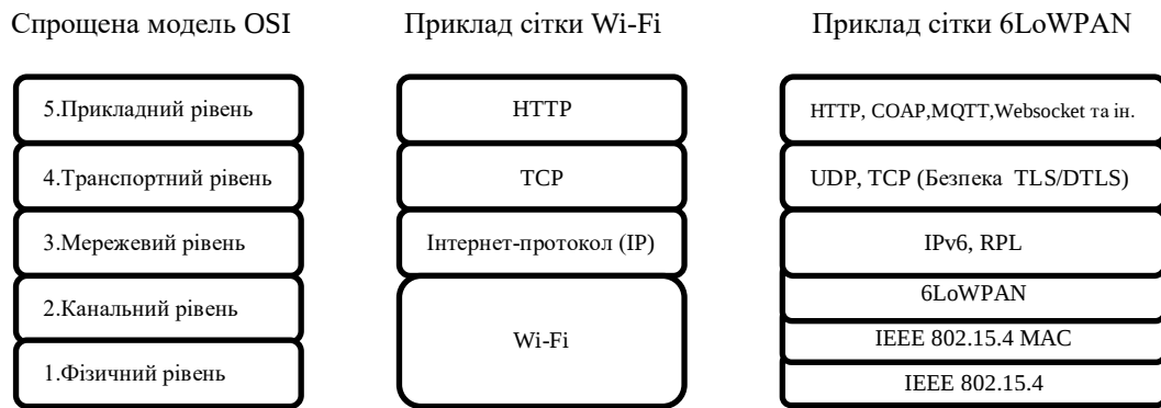
Рис. 3.16. Приклади моделі OSI, стеків Wi-Fi та 6LoWPAN
