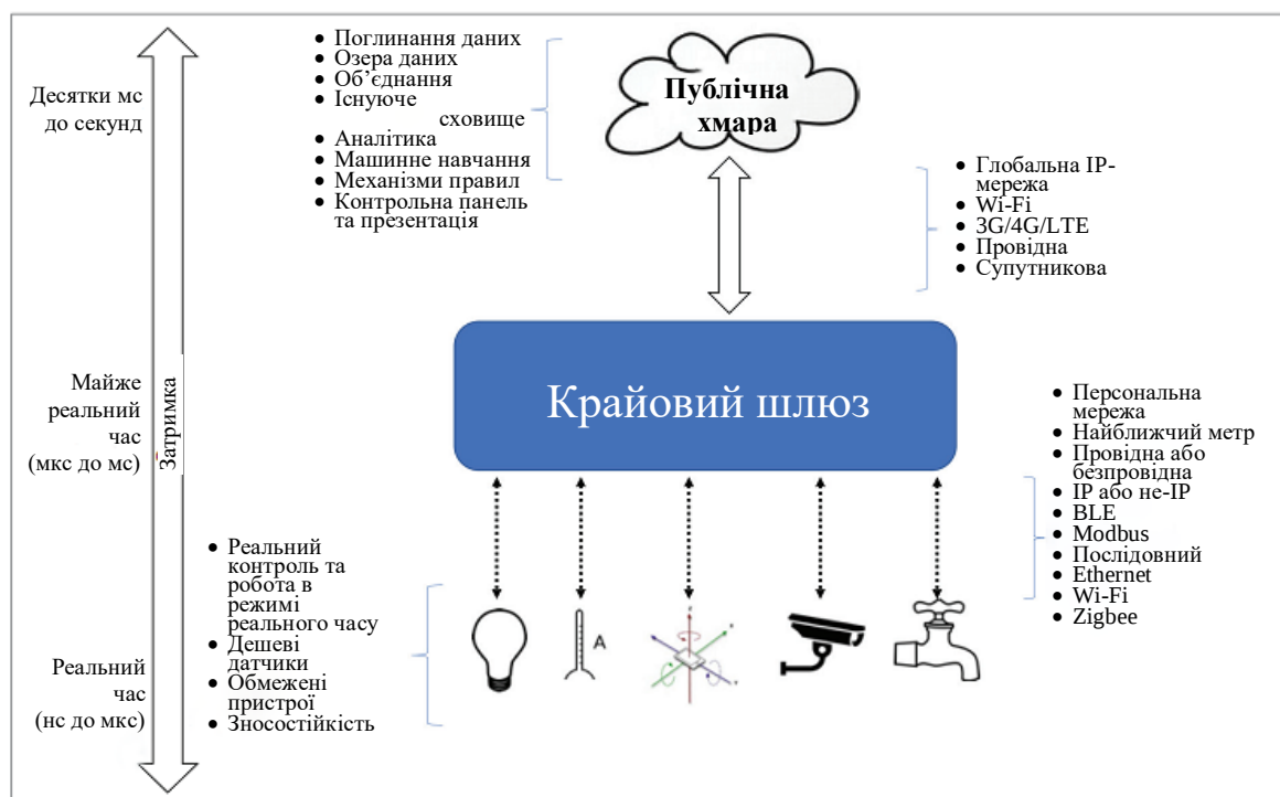
Рис. 4.4. Ефекти затримок в хмарі. Реакція в реальному часі має вирішальне значення в багатьох додатках IoT і змушує пересувати обробку ближче до кінцевого пристрою [1]
