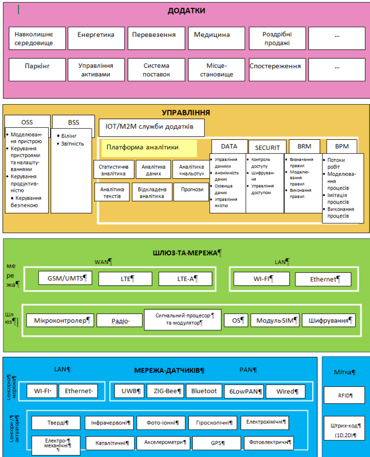
Рис. 1.9. Архітектура IoT
