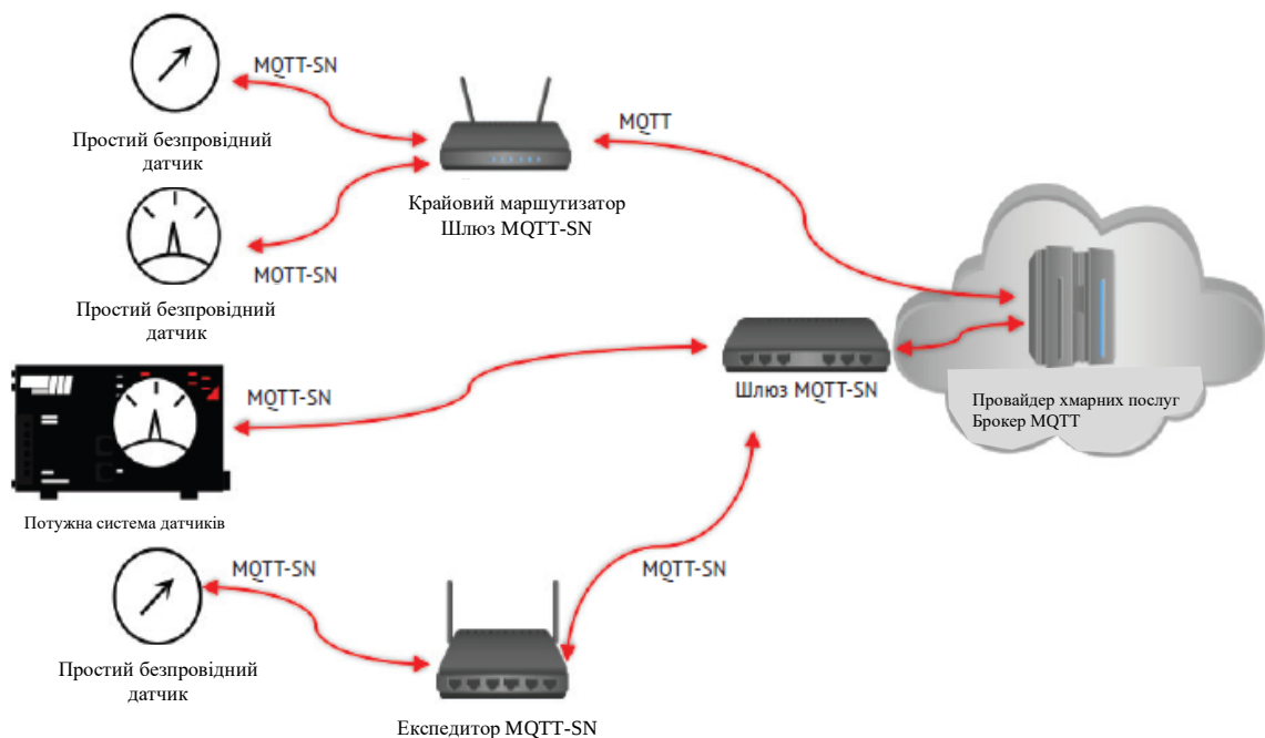
Рис. 3.29. Топологія MQTT-SN
