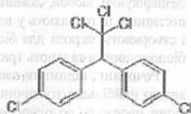
Рис. 11.1. Структура дихлордифеніл-трихлоретану.
