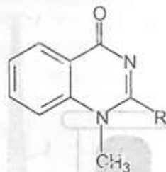
Рис. 7.12. Структура гломерину.
