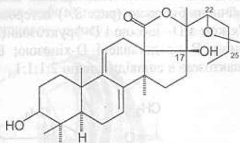
Рис. 8.5. Структура 22,25-оксидоголотуриногеніну.
