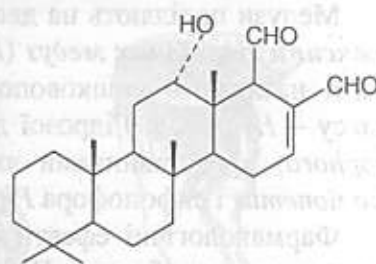
Рис. 6.4. Структура токсину деацетилскаларідіал.
