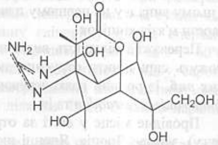
Рис. 8.10. Структура тетродотоксину.
