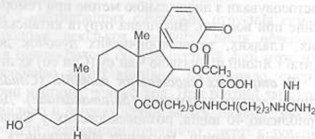
Рис. 9.4. Структура буфотоксину.
