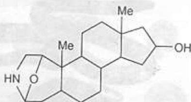
Рис. 9.7. Структура самандарину.
