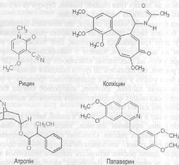
Рис. 6.10. Структура алкалоїдів.
