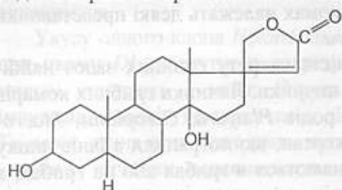
Рис. 7.10. Структура узарегину.
