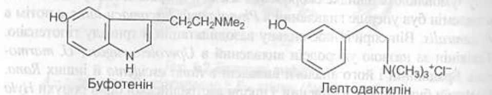
Рис. 9.3. Структура токсинів жаб.
