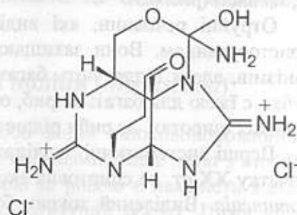
Рис. 6.2. Структура саксітоксину.
