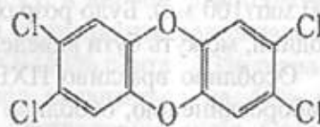
Рис. 11.4. Структура діоксину.
