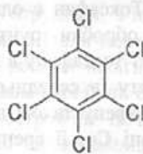
Рис. 11.2. Структура гексахлорбензолу.
