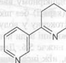
Рис. 6.6. Структура анабазеїну.
