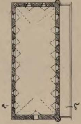
Планъ здания одинаковой для двухъ эржей рис. 90
