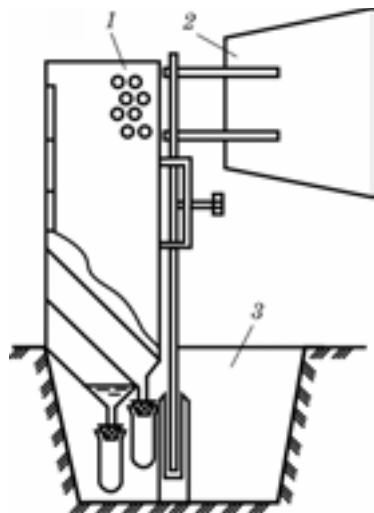
Рис. 13. Пиловловлювач УПЗ-50
