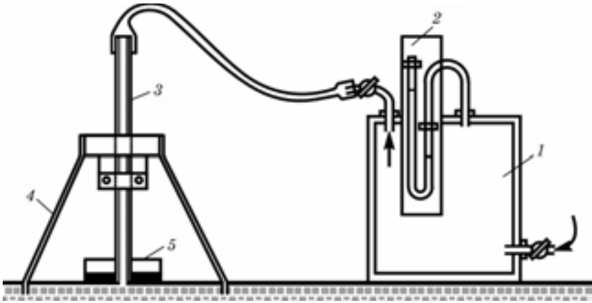
Рис. 8. Прилад Еванса та Кірхама
