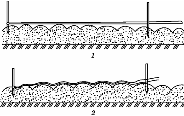
Рис. 73. Вимірювання гребенястіості оранки 10-метровим шнуром
