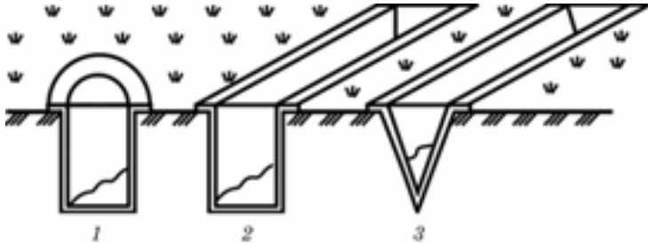
Рис. 11. Вловлювачі ґрунту:
